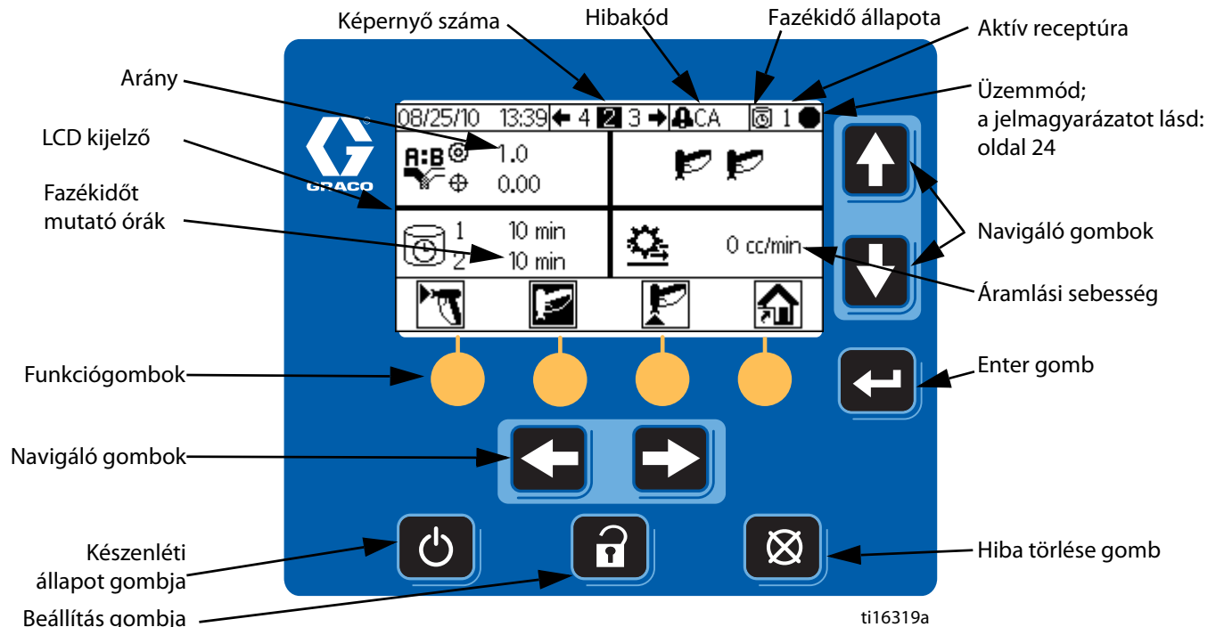
ÁBRA 10. Kijelzőmodul
