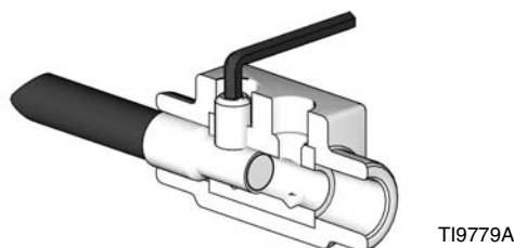
FIG. 9: Serraggio della vite di arresto
