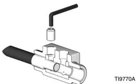
FIG. 8: Inserimento del filo e della vite di arresto
