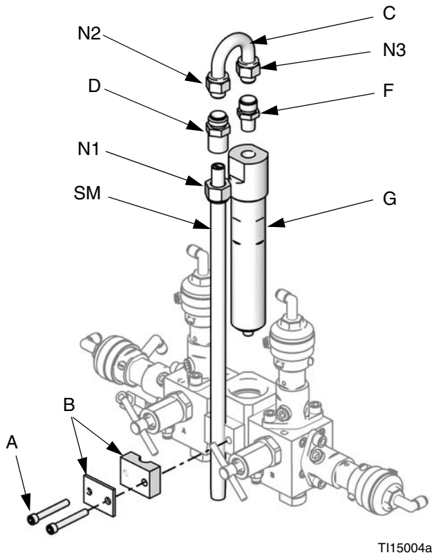
FIG. 8 Smontare l'integratore e il miscelatore statico
