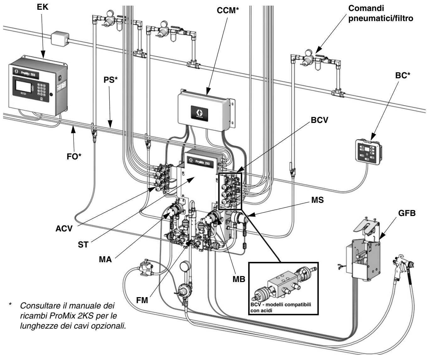
FIG. 2 Sistema manuale, illustrato con dosatore G3000, cambio colore/catalizzatore, una scatola lavaggio pistola e dosatore del solvente accessorio
