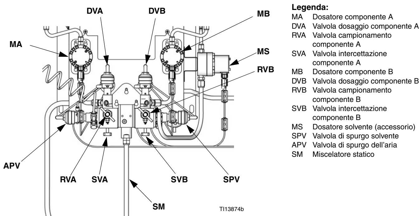
FIG. 10 Stazione del fluido per montaggio a parete, dosaggio dinamico
