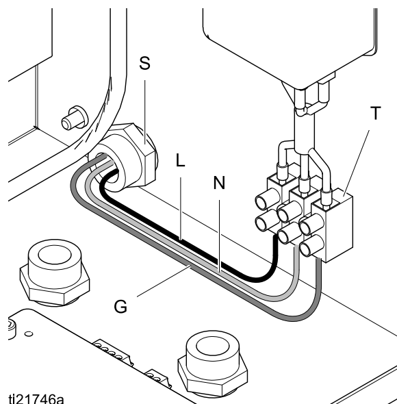
ti21746a Figure 21 コントロールボックスの電気接続
