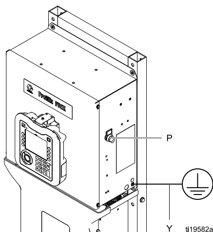
Figure 22 接地ネジと電源スイッチ
