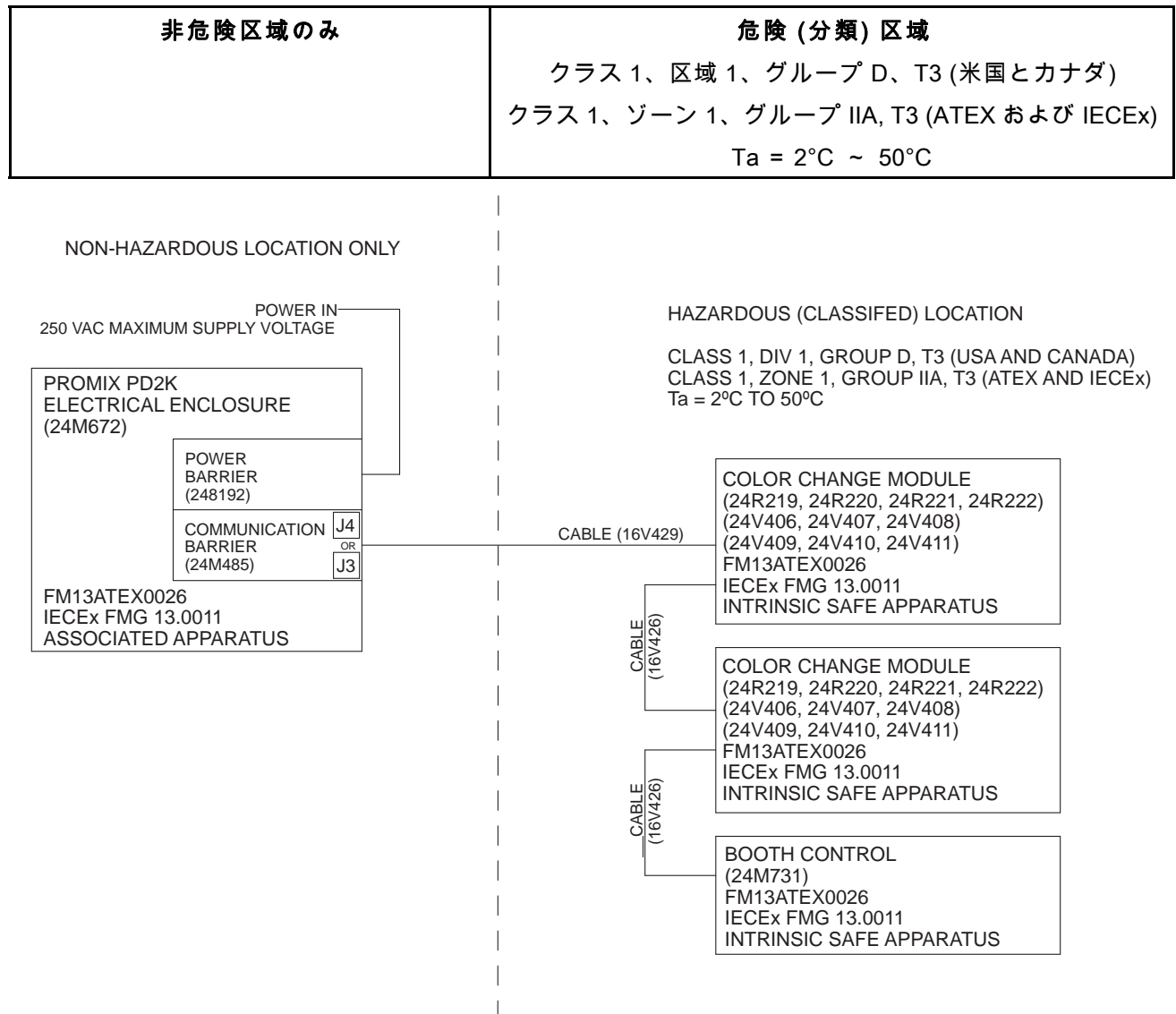
Figure 8 システムコントロール図面 16P577
