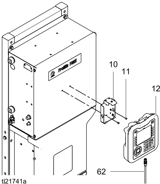
Figure 12 ディスプレイ モジュールの取り付け
