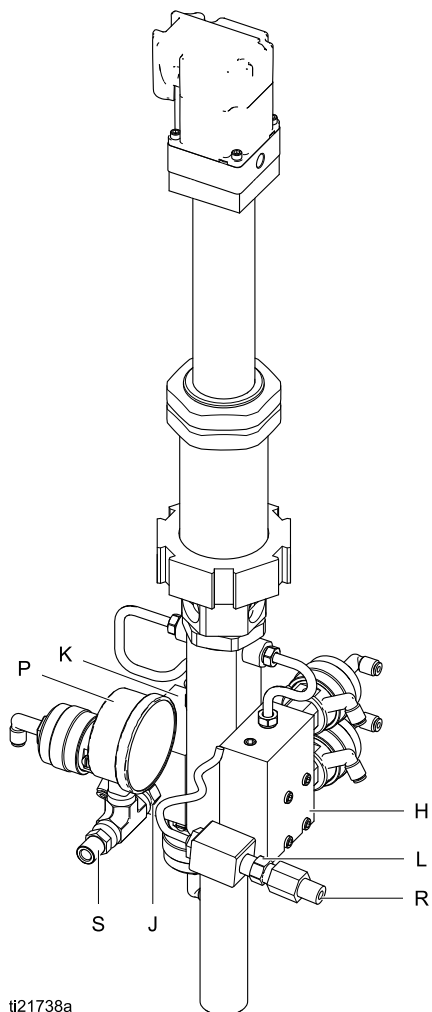
Figure 18 ポンプのインレットとアウトレット接続
