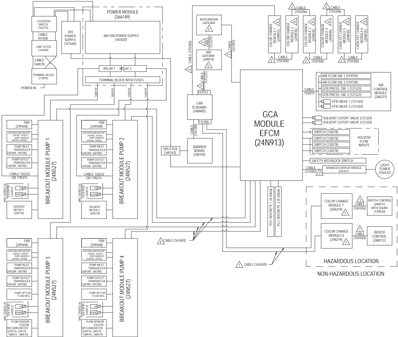
Figure 30 電気回路図、シート 1
