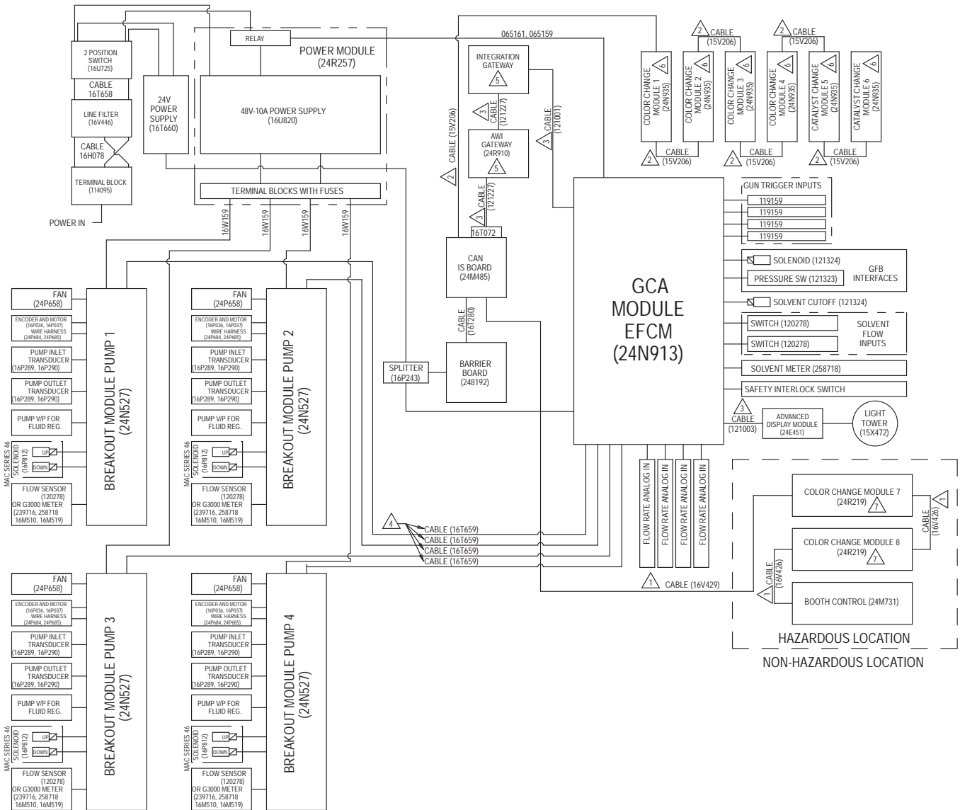
Figure 24 電気回路図、シート 1
