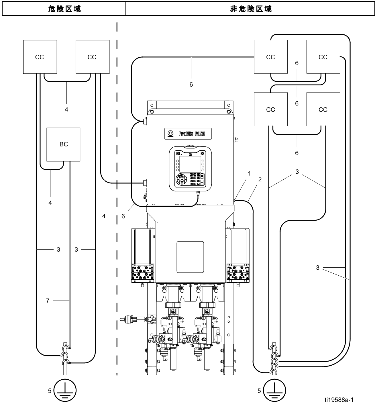
Figure 23 システムの接地
