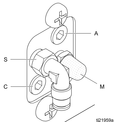
Figure 17 エアマニホールドの接続 キー
