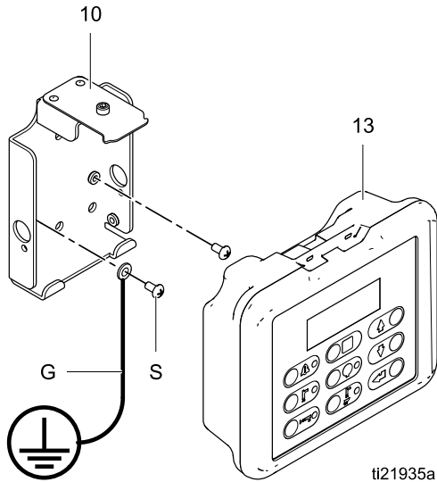
Figure 14 ブース コントロール ブラケットの接地
