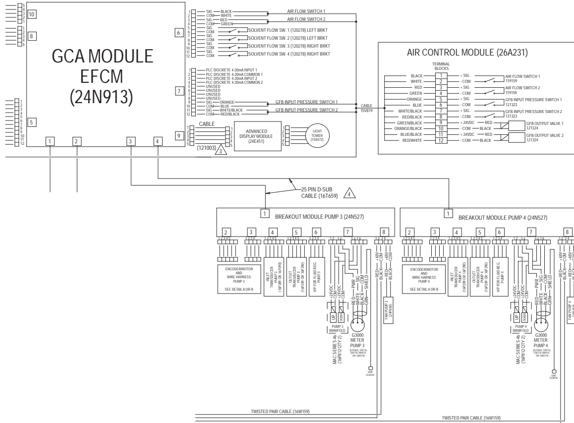
Figure 32 電気回路図、シート 2、パート 2
