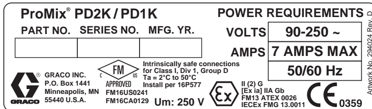
Figure 2 24M672 & 26A188 制御ボックス識別ラベル
