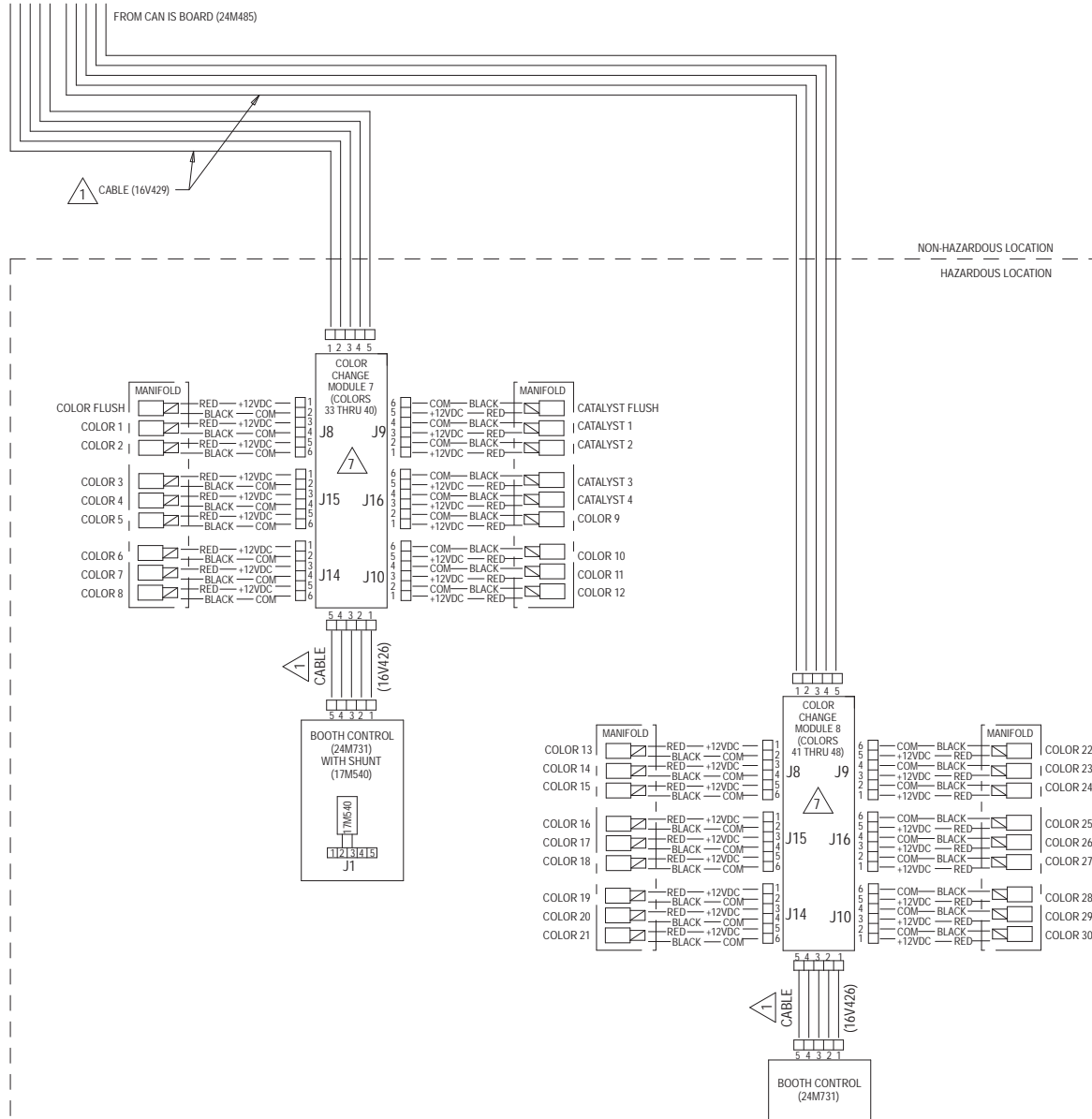
Figure 34 電気回路図、シート 3、パート 2
