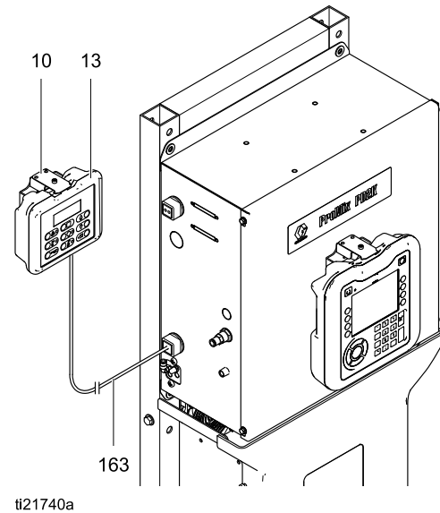
Figure 15 ブース コントロールの設置
