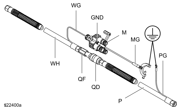
ti22400a Figure 20 静電エアホースクイック取り外しキット
