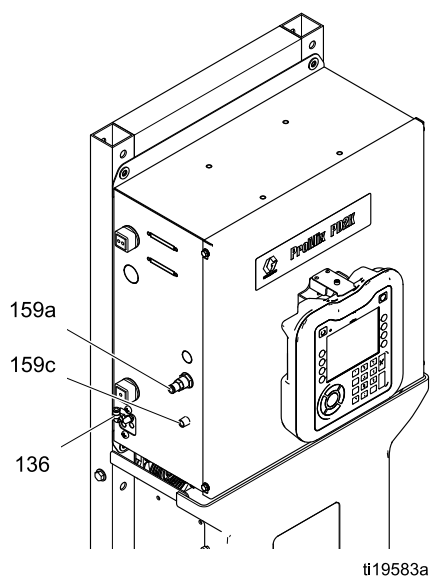
Figure 16 噴霧空気の接続
