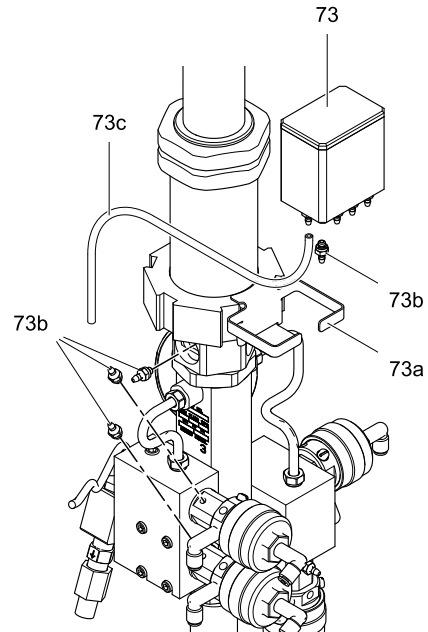
Figure 19 TSL カップ キットの取り付け
