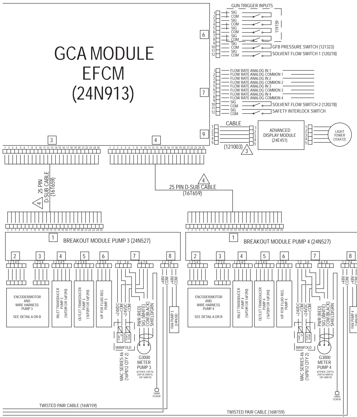
Figure 26 電気回路図、シート 2、パート 2
