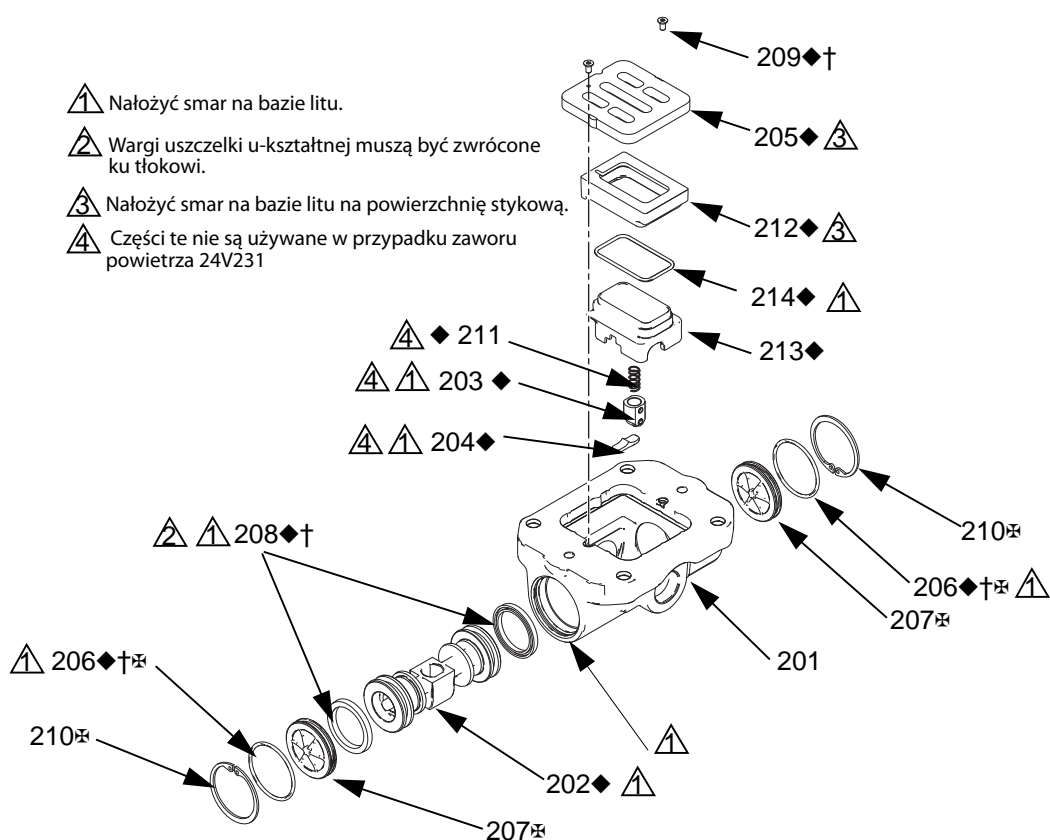
Rys. 2. Zespół zaworu powietrza
