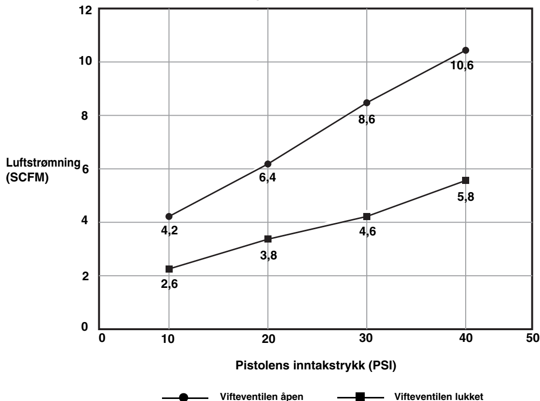
Luftstrømning, standard AA-serien luftkappe
