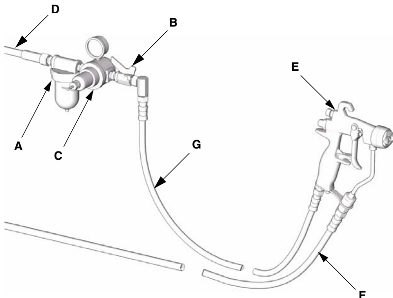
FIG. 1: Typisk monteringsanvisning (Modell G15 er vist)
