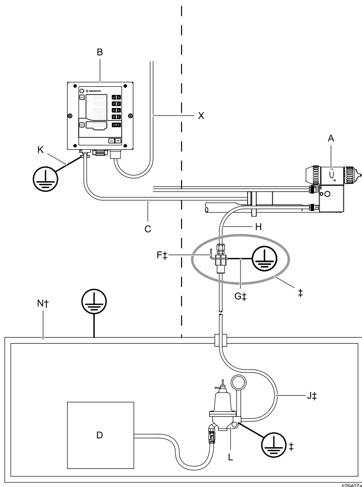
일반 설치(무통합)
