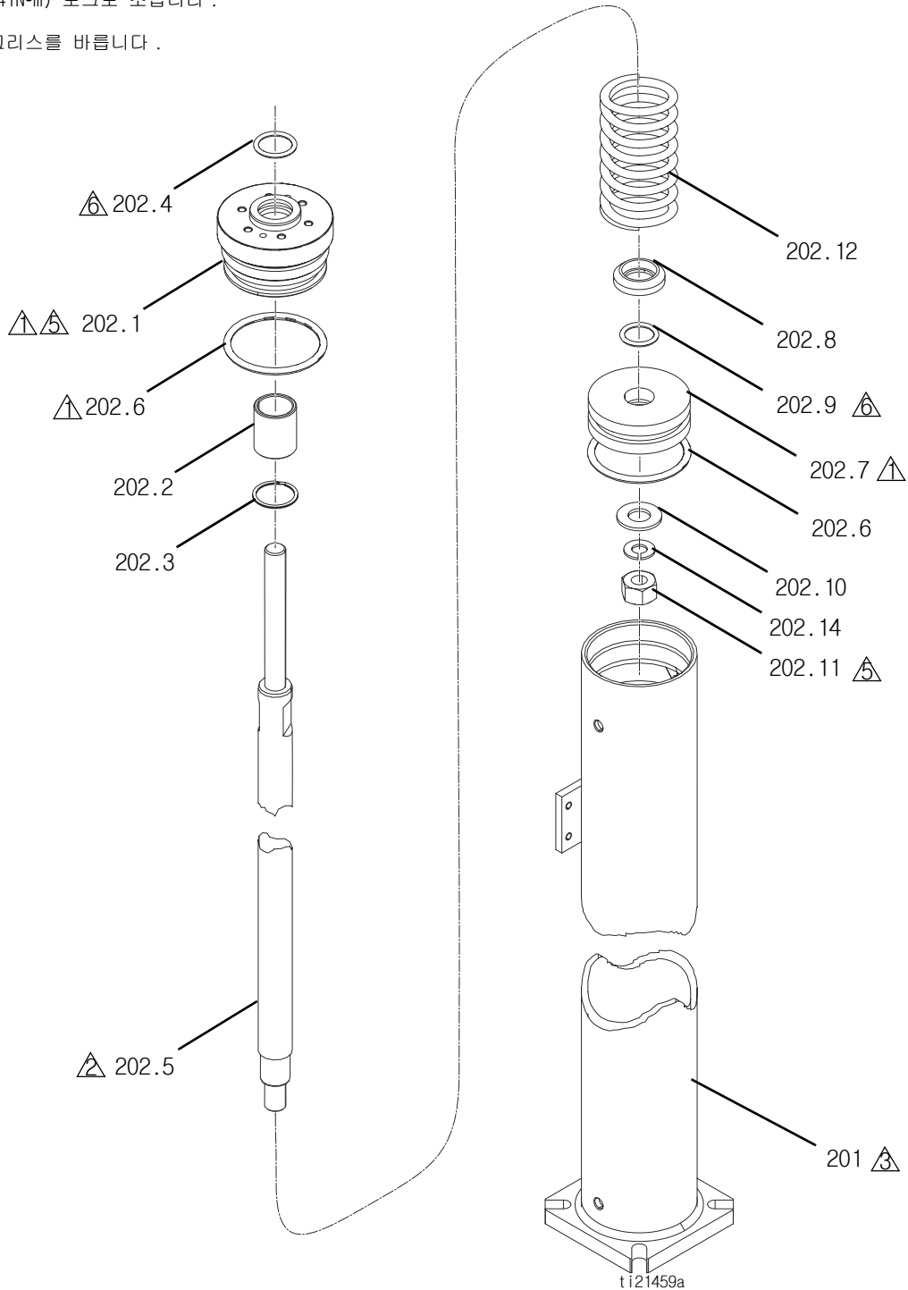
그림 5: 55 갤런 공기 실린더
