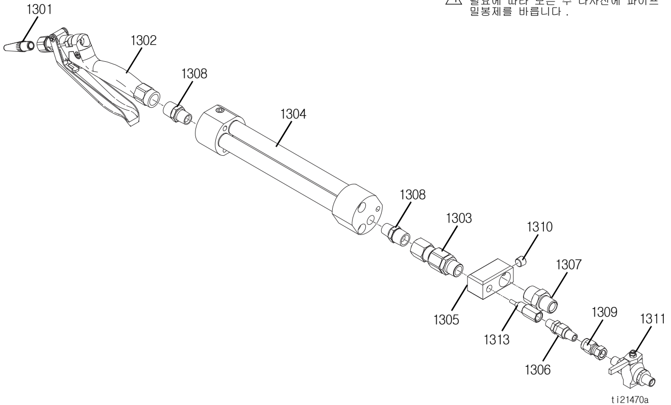
그림 16: Ultra-Lite TriCore
