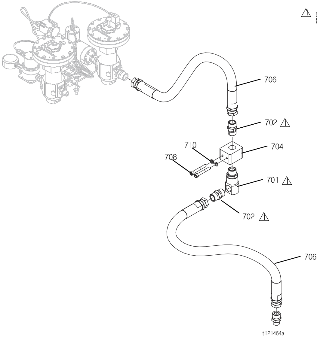
그림 11: 고용량 호스
