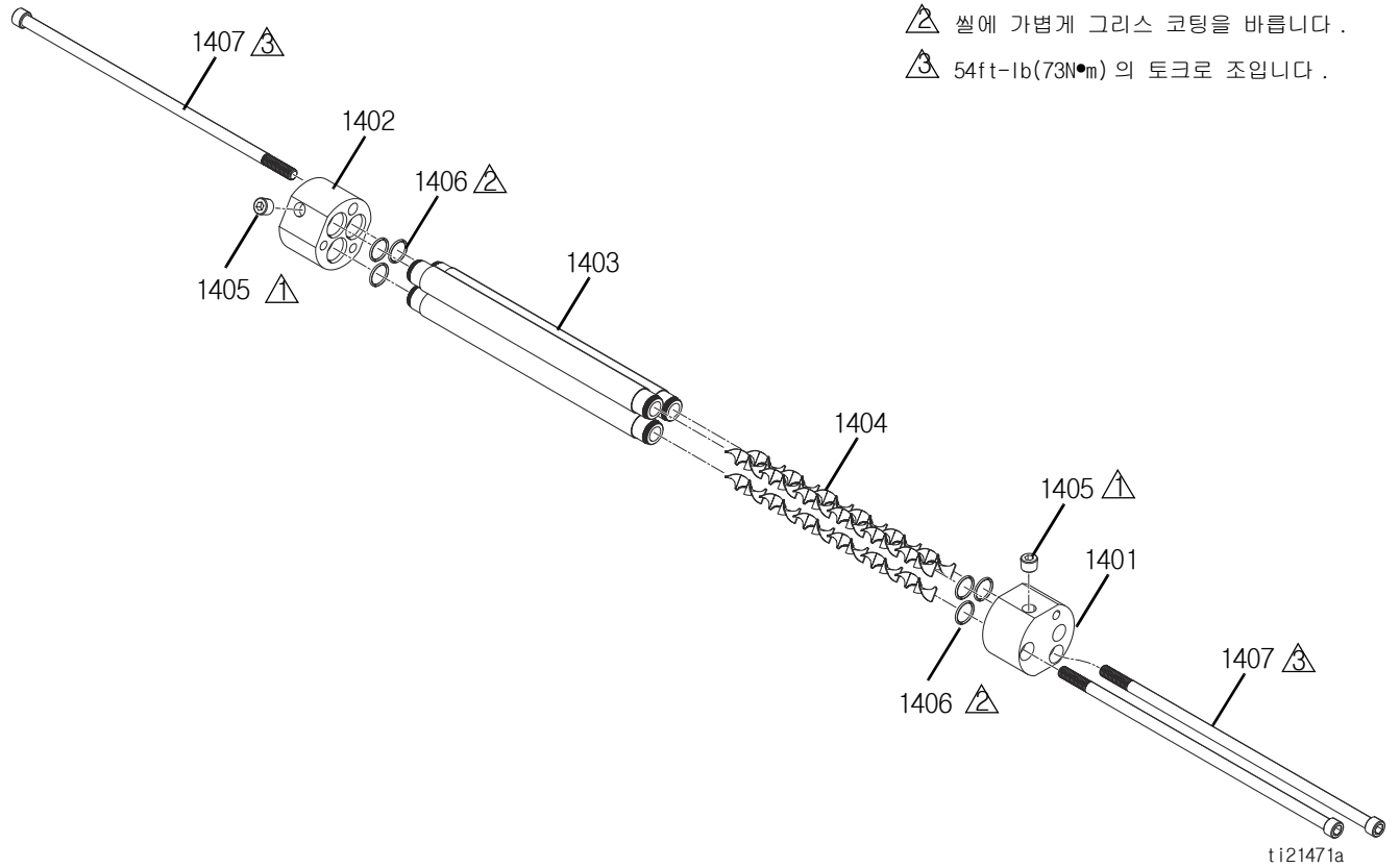
그림 17: Tri-Core 혼합기
