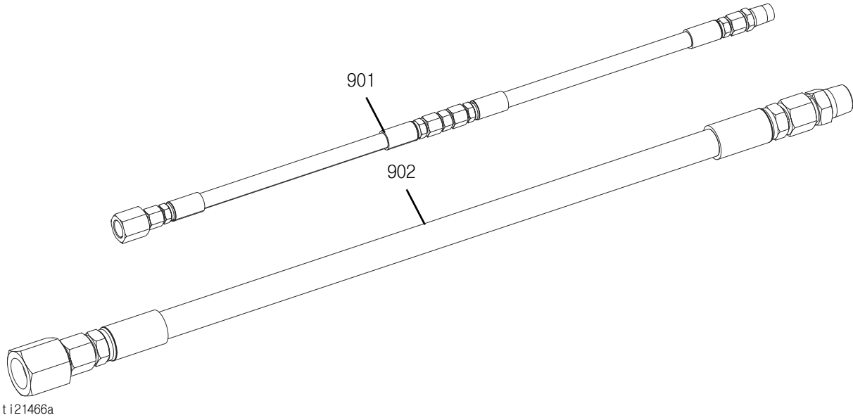
그림 13: 호스 키트
