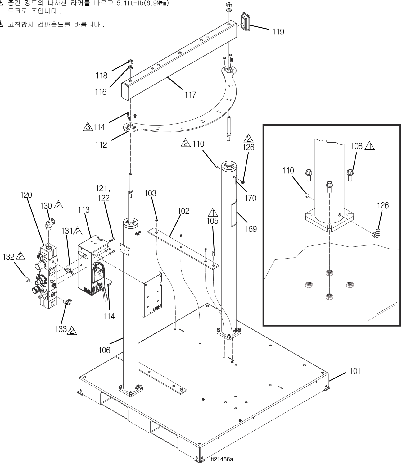
그림 2: 베이스
