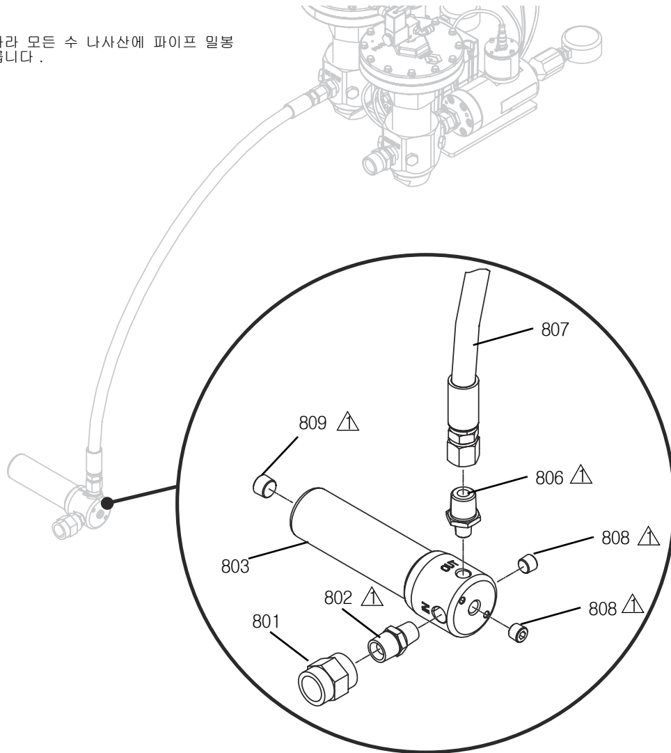
그림 12: 저용량 호스
