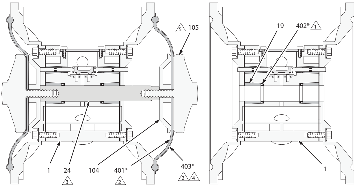
04708 Genomskäring med membranerna på plats
