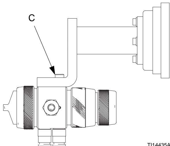
Pistolets sans collecteur
