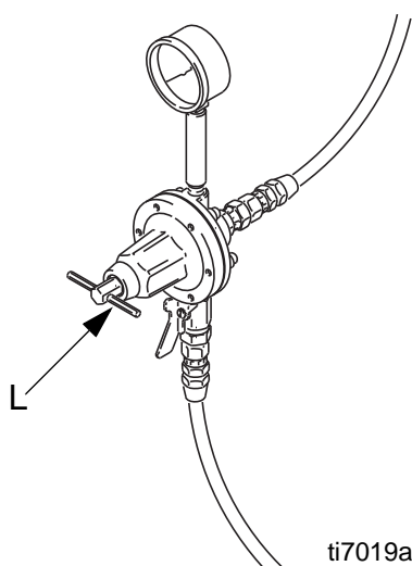
Fig. 11 : Régulateur de pression du fluide
