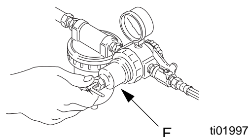
Fig. 12 : Régulateur de pression d'air
