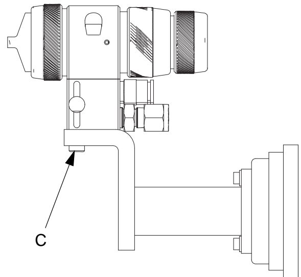
Pistolets avec collecteur
