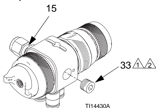
FIG. 2 : Pistolets sans collecteur
