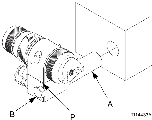
FIG. 3 : Montage du bras à mouvement alternatif
