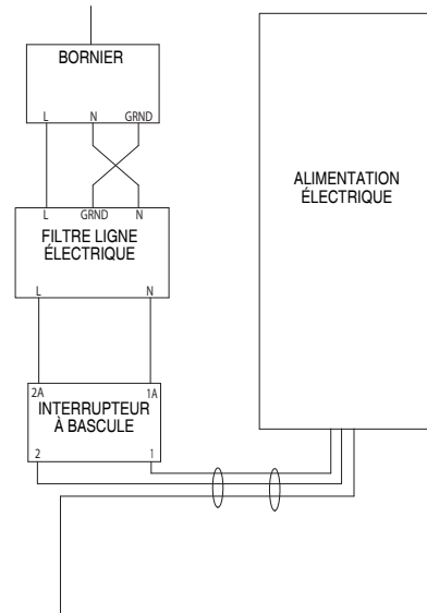
FIG. 10. Schéma électrique
