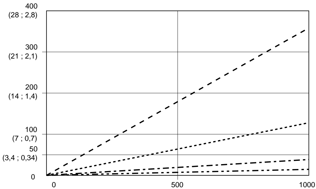
Fig. 59. Performances du dosage dynamique (rapport 5:1, produit 90 centipoises, pression côté A 100 psi)
