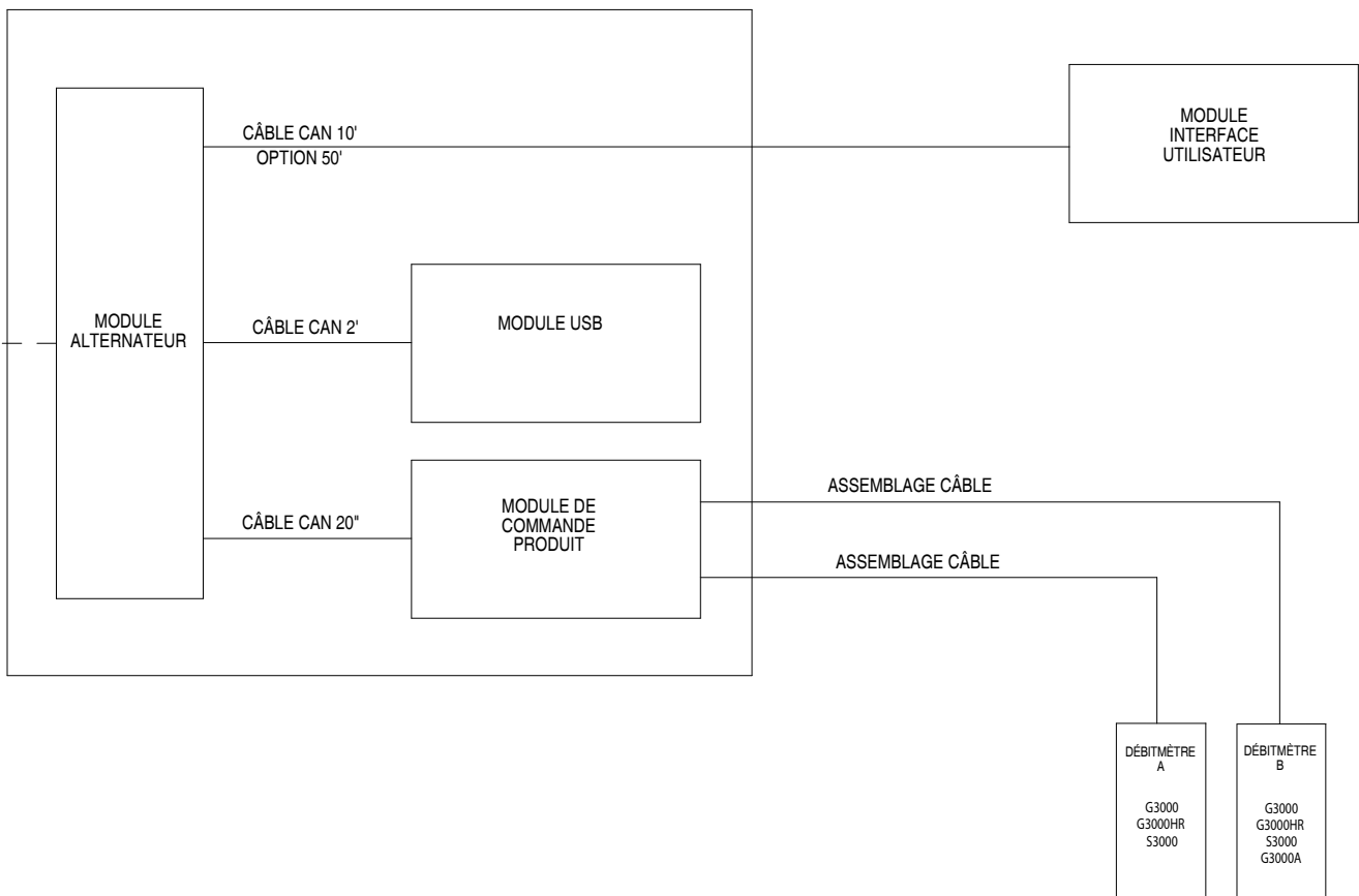
FIG. 1. Installation sur sites à risque
