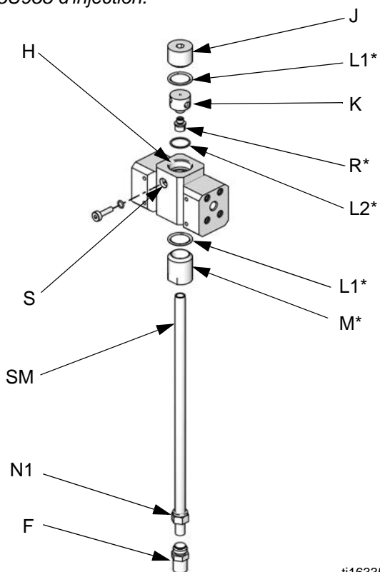
FIG. 8. Installation du kit 15U955 d'injection
