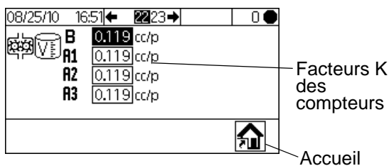
Fig. 46. Calibrage 1 (écran 22)
