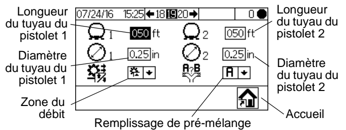
Fig. 40. Configuration 2 (écran 19)
