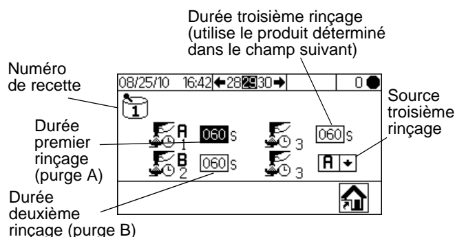
FIG. 44. Recette 1-2 (écran 29)
