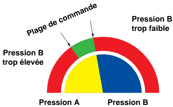
FIG. 53. Plage de commande A/B avec un limiteur correctement dimensionné
