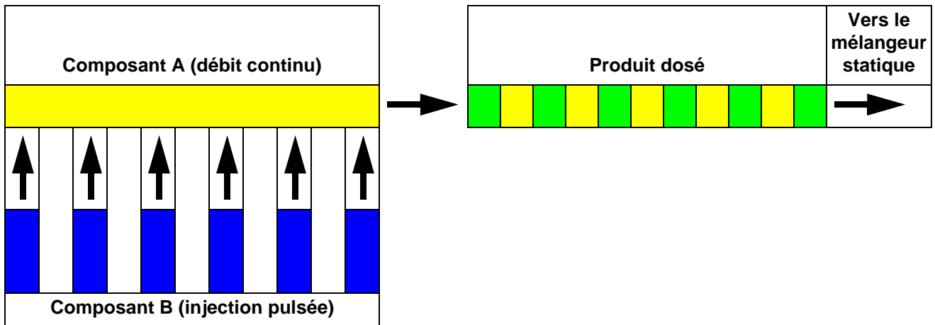
FIG. 55. Schéma de principe du fonctionnement du dosage dynamique
