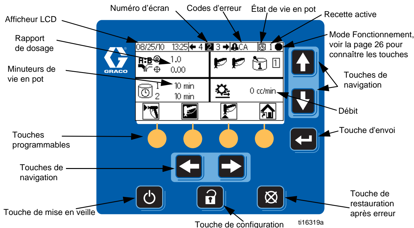
FIG. 13. Module d'affichage
