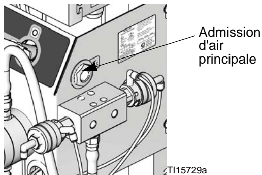
FIG. 3. Raccordement d'air principal
