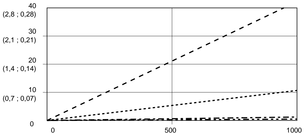
Fig. 60. Performances du dosage dynamique (rapport 30:1, produit 90 centipoises, pression côté A 100 psi)
