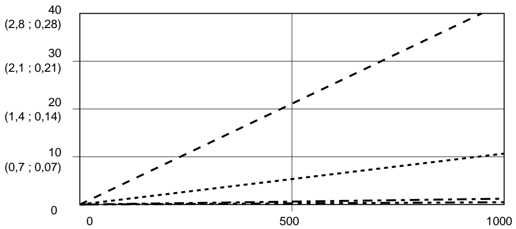
Fig. 62. Performances du dosage dynamique (rapport 30:1, produit 90 centipoises, pression côté A 100 psi)
