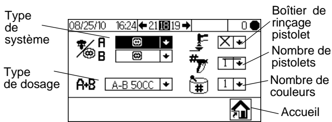
Fig. 38. Configuration 1 (écran 18)
