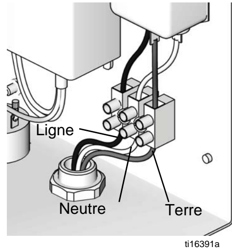
FIG. 9. Branchements électriques du boîtier de commande
