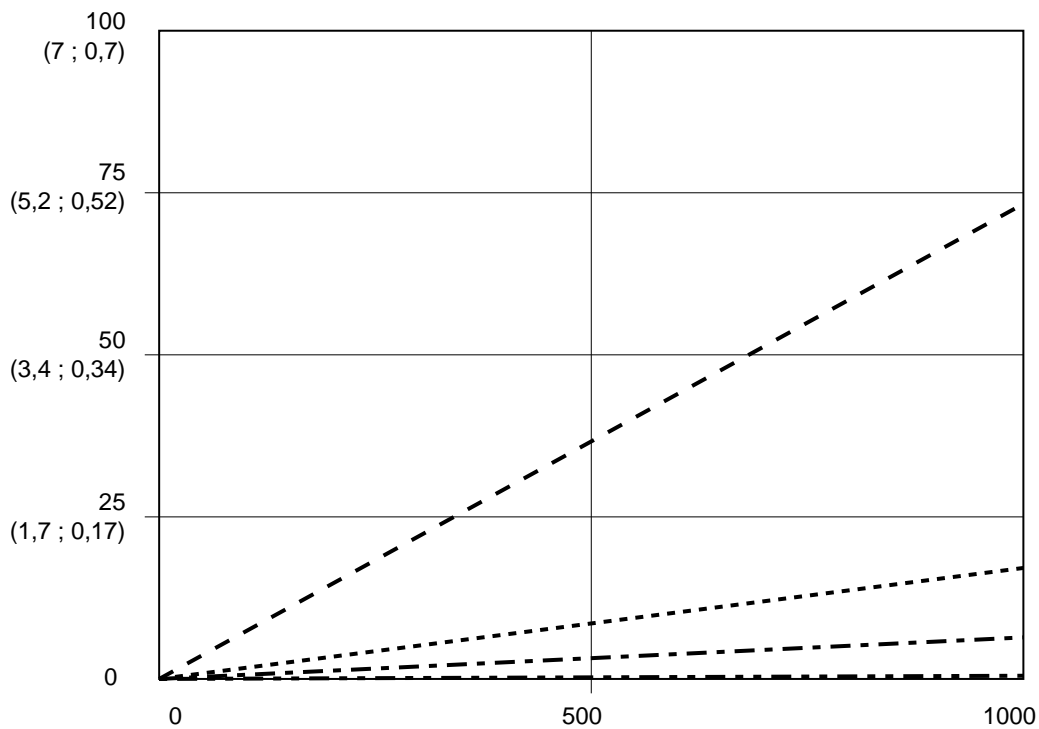
FIG. 61. Performances du dosage dynamique (rapport 20:1, produit 90 centipoises, pression côté A 100 psi)
