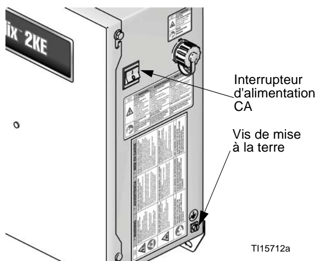
Fig. 11. Vis de terre et interrupteur électrique
