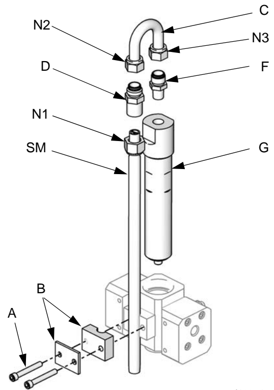
FIG. 7. Démontage de l'intégrateur et du mélangeur statique
