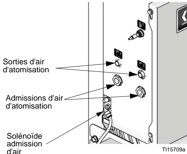
FIG. 4. Raccordement d'air d'atomisation
