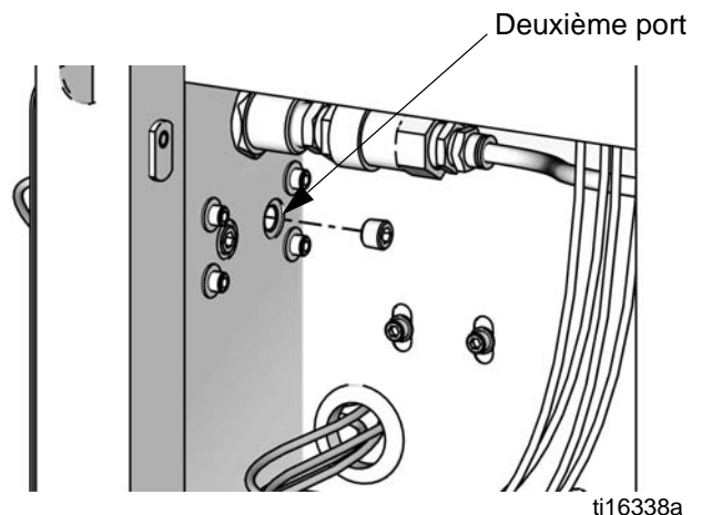
FIG. 5. Port de recirculation de peinture
