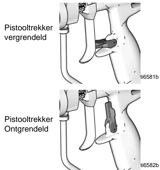
FIG. 5. Veiligheidspal pistool
