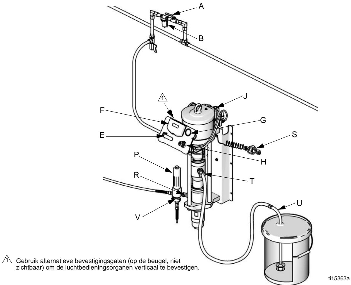
FIG. 2: Voorbeeldinstallatie van een wandconsole
