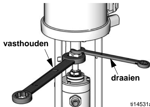
FIG. 7. Draai de koppelmoer los.
