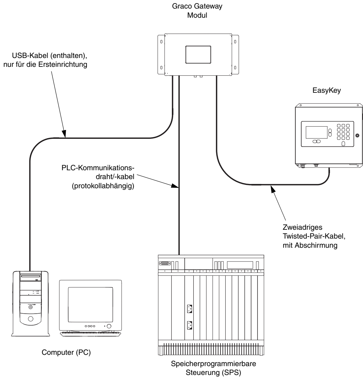
ABB. 1: Typische Installation Graco Gateway
