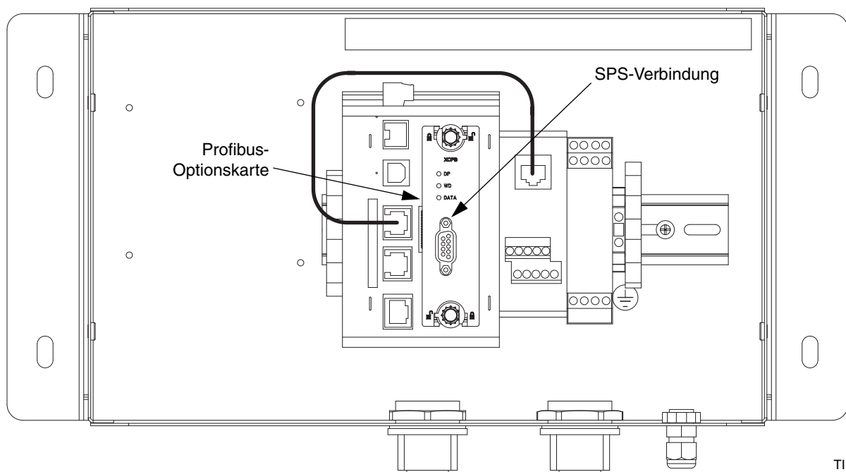
ABB. 47: Profibus-SPS-Verbindung
