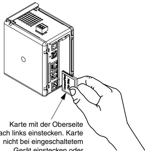
ABB. 11: CompactFlash-Karte installieren
