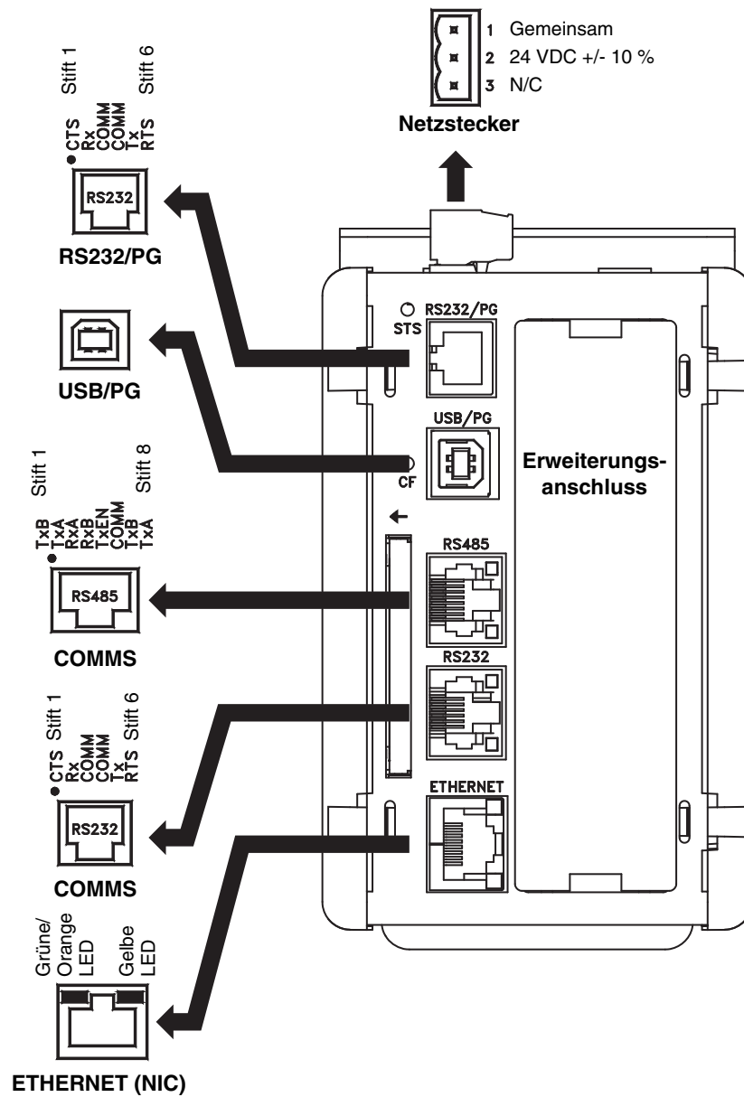
ABB. 4: Graco Gateway-Anschluss – Kontaktstifte
