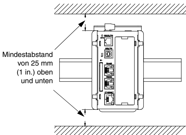
ABB. 10: Steuerung an einer DIN-Schiene befestigen
