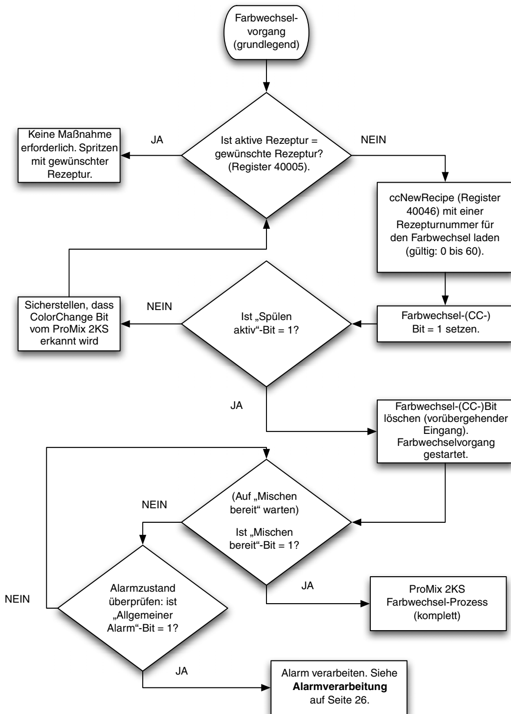
ABB. 28: Flussdiagramm zum Farbwechselfvorgang
