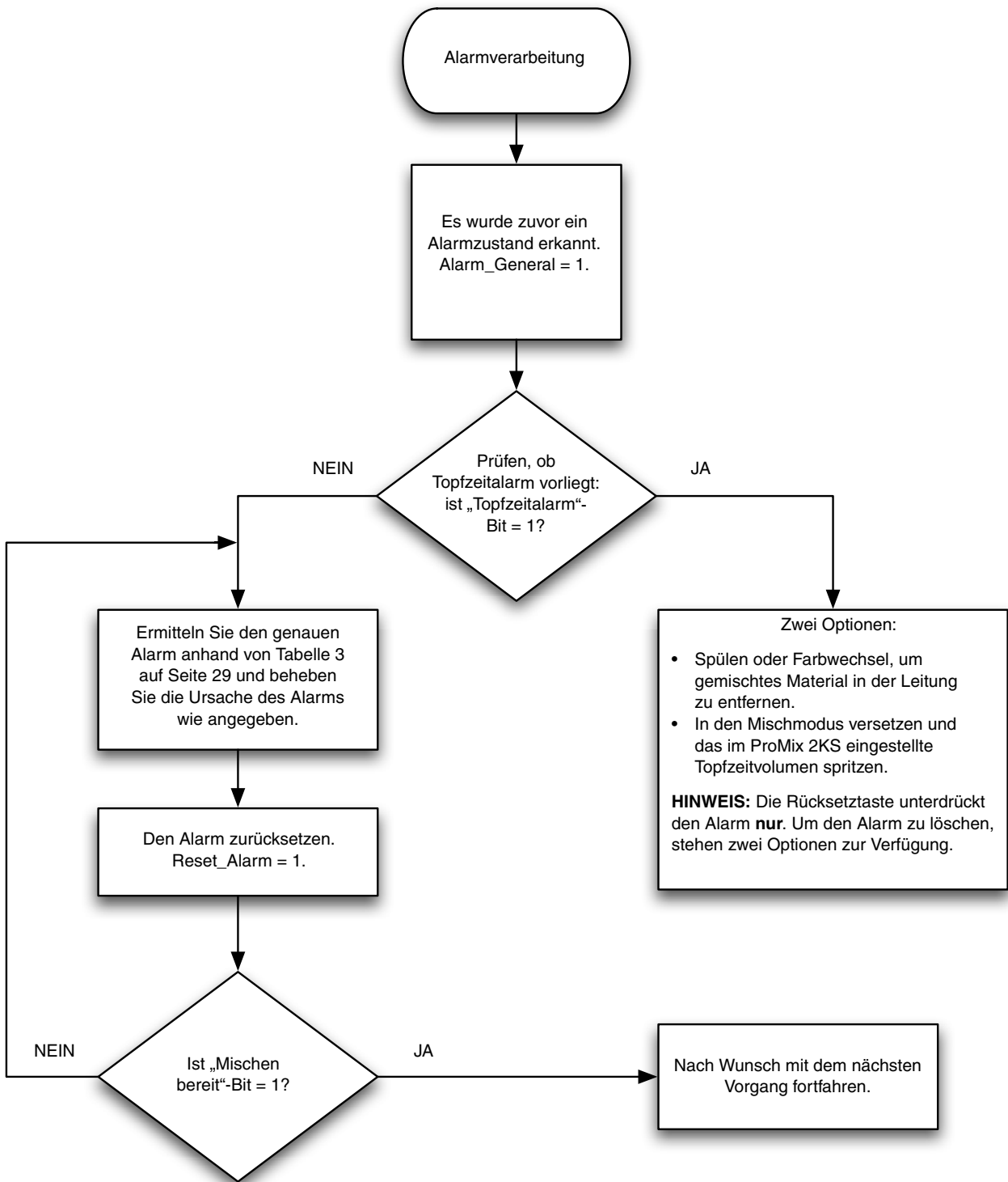
ABB. 29: Flussdiagramm zur Alarmverarbeitung
