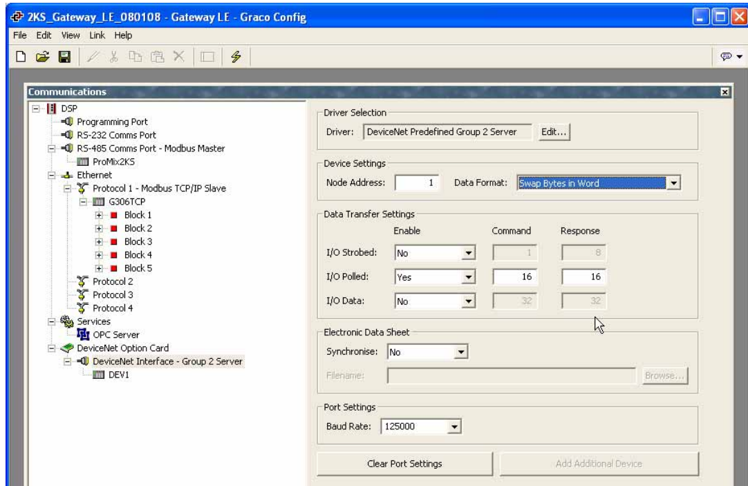
ABB. 33: Geräteeinstellungen
