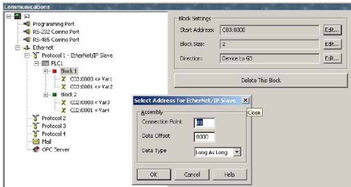
ABB. 74. Ethernet-Blockeinstellungen
