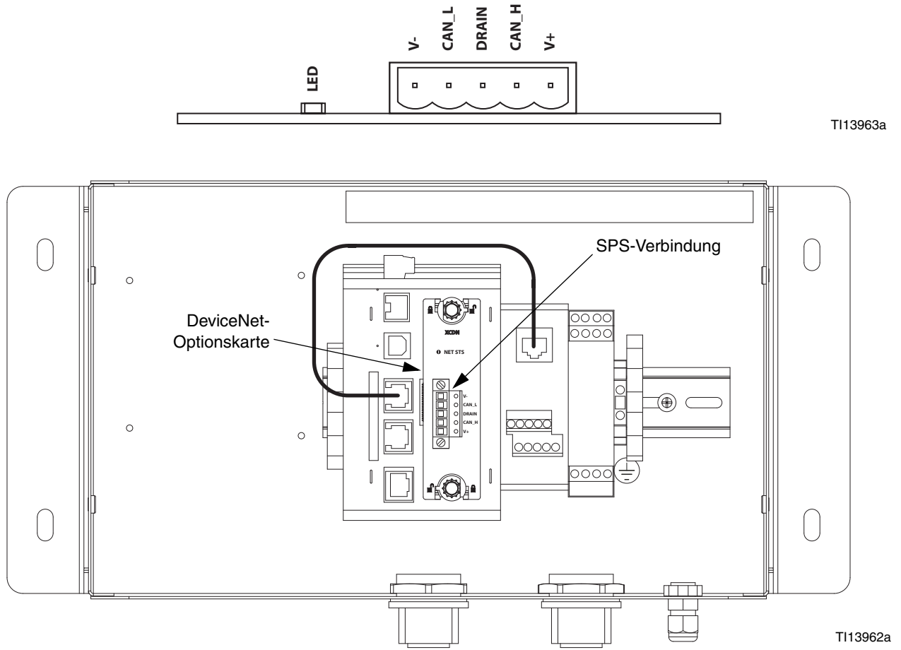
ABB. 30: Kontaktstifte des DeviceNet-Anschlusses und SPS-Verbindung
