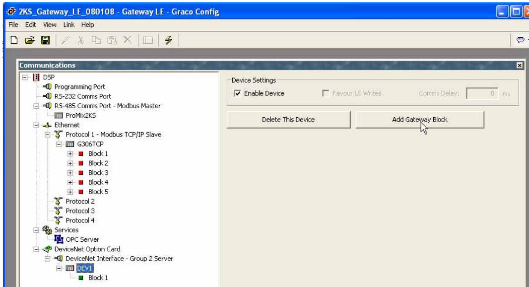
ABB. 34: Gateway-Block hinzufügen
