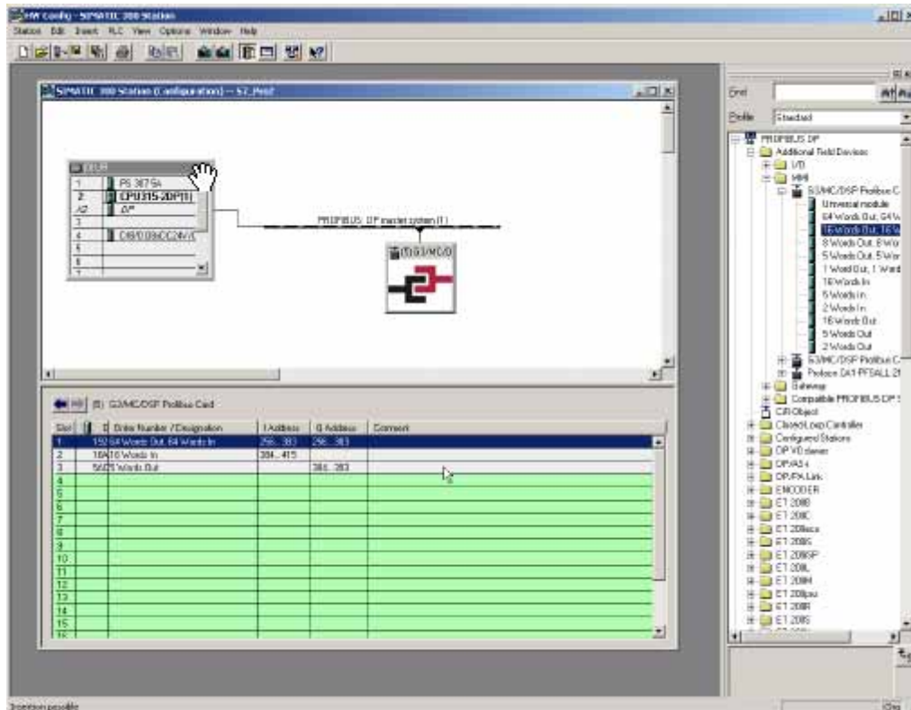
Abb. 58: Datenblöcke konfigurieren
