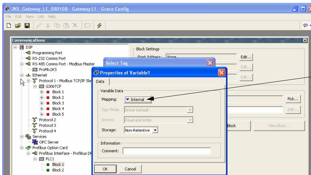
ABB. 63: Variableneigenschaften
