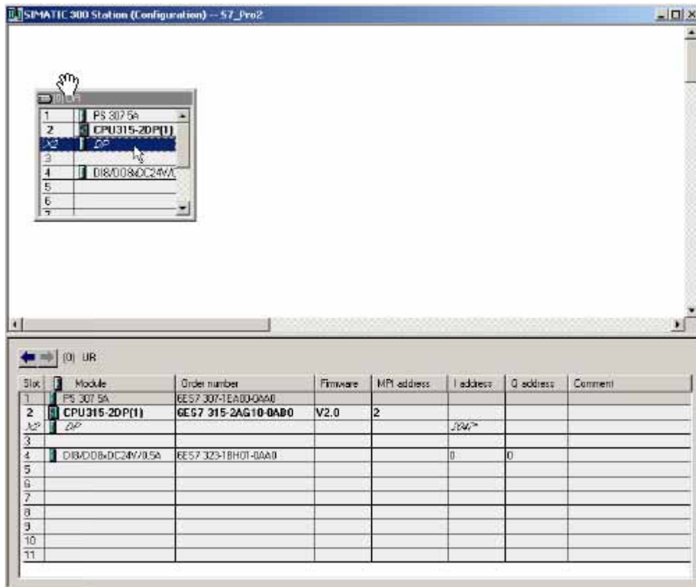
ABB. 52: DP-Eigenschaftsfenster
