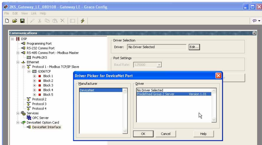
ABB. 32: DeviceNet-Server auswählen
