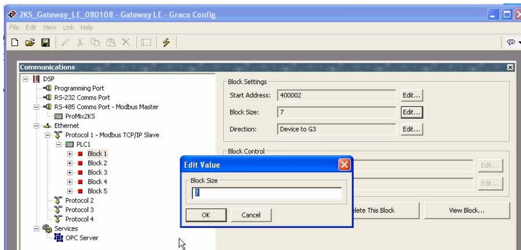
ABB. 23: Blockgröße festlegen
