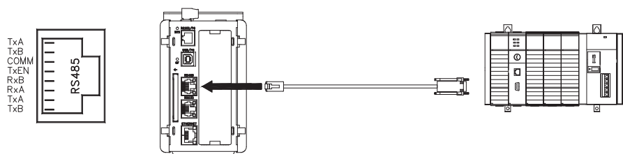
ABB. 5: RS485-Kommunikationsanschluss (Typische ProMix 2KS-Verbindung)
