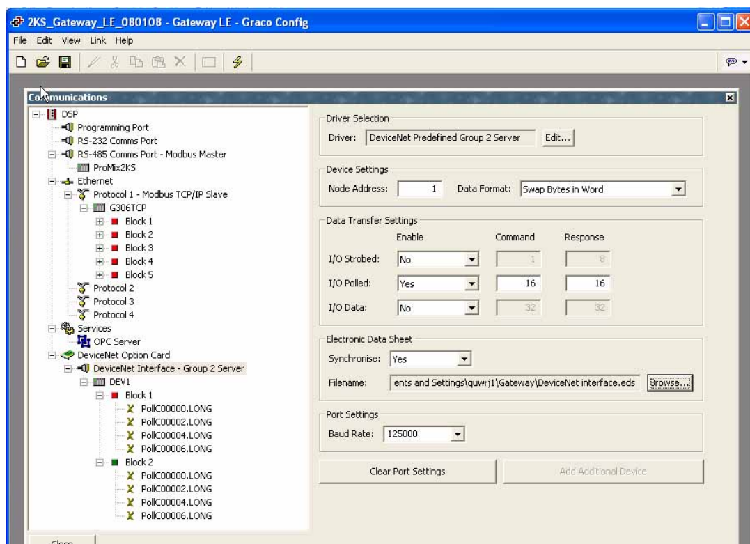
ABB. 37: Automatische EDS-Aktualisierung
