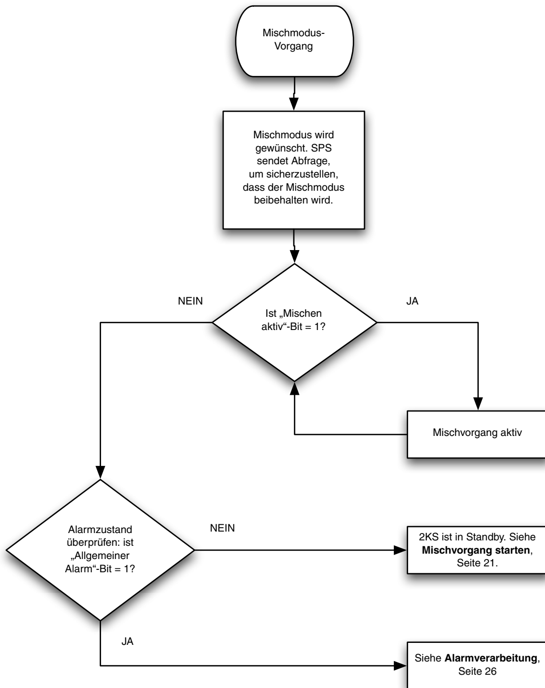
ABB. 26: Flussdiagramm zum Mischmodus-Vorgang
