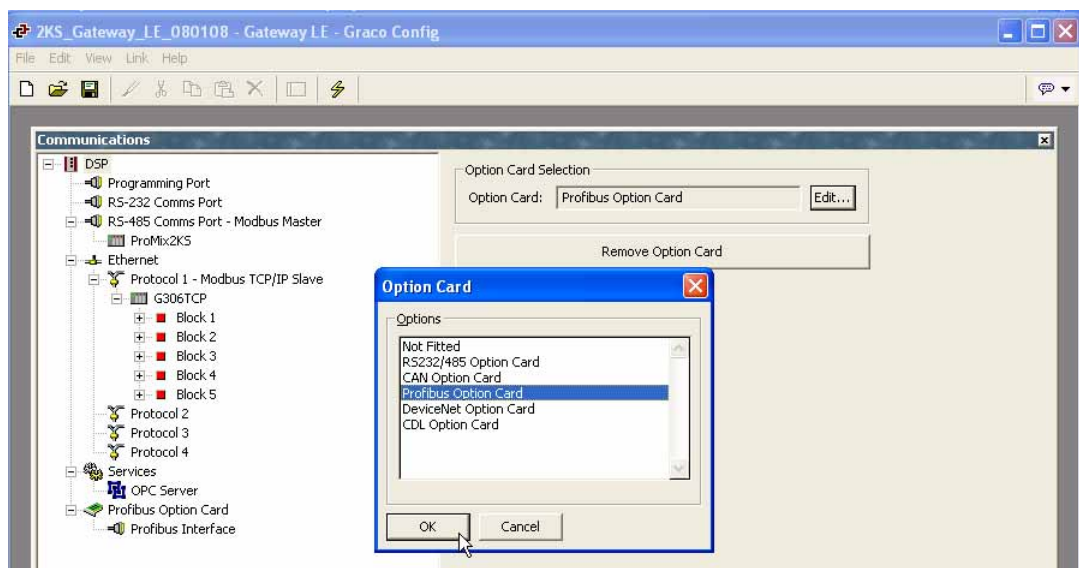
ABB. 59: Profibus-Optionskarte auswählen
