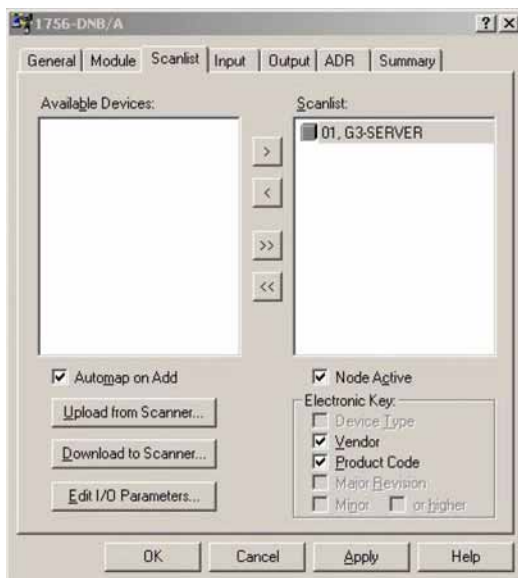
ABB. 43: DeviceNet-Master konfigurieren
