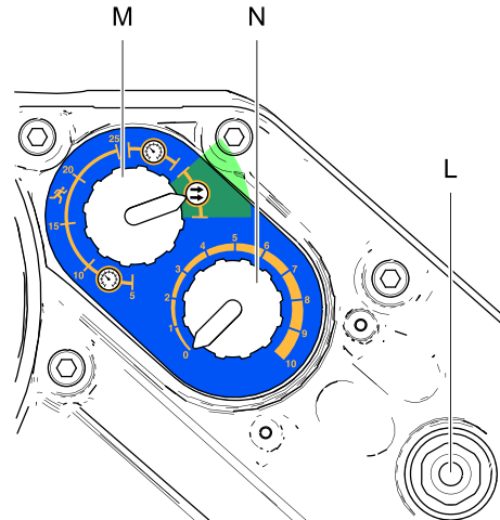
Figure 13 Debietmodus
