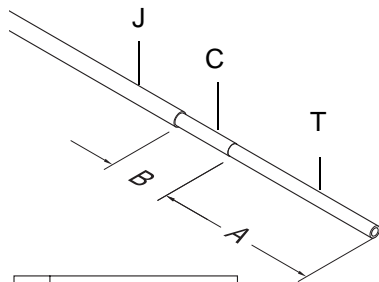
Fig. 8 Dimensiones de la manguera con carcasa en el recinto WB100
