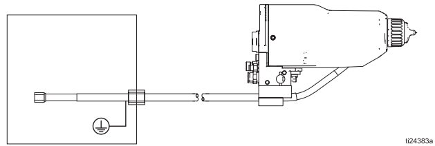
Fig. 10 Conexión de la manguera de fluido con carcasa a un recinto aislado de otra marca
