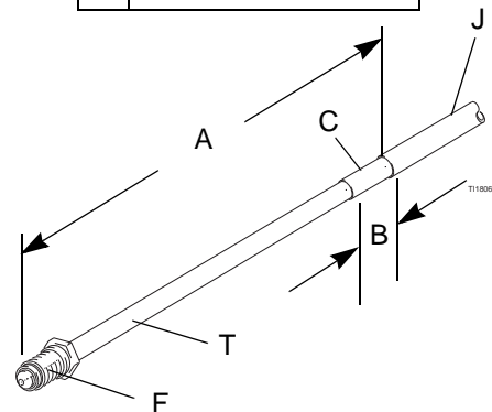
FIG. 6. Dimensiones de la manguera a base de agua
