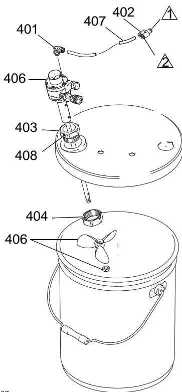
Fig. 13 Kit agitador 245895
