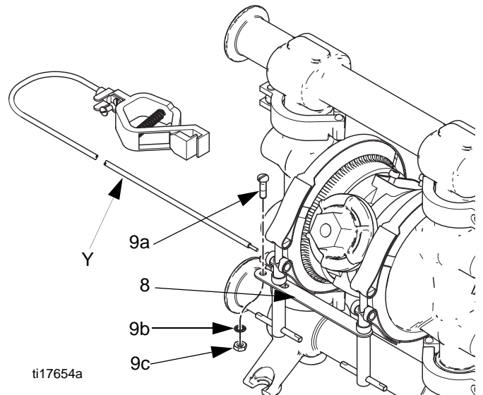
FIG. 1: Messa a terra della pompa
