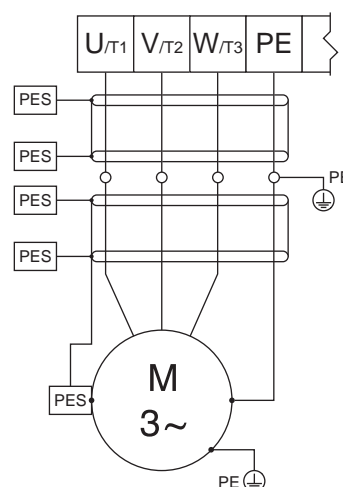
Figure 7 Draadverbindingen van de motor naar de VFD
