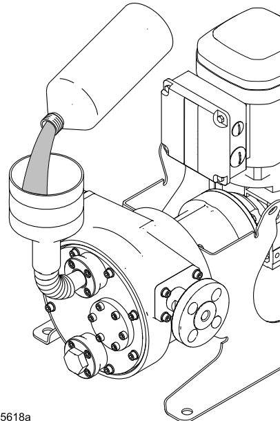
Figure 4 Vul de pomp met slangsmoermiddel
