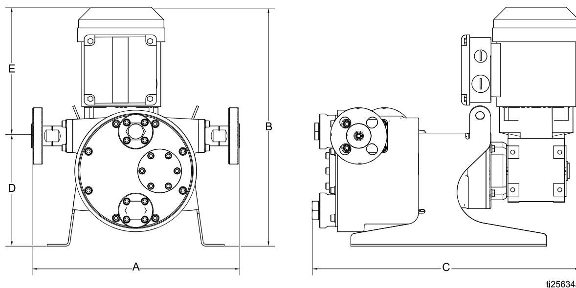
Figure 18 Wisselstroompompen ST10, ST23, en ST30
