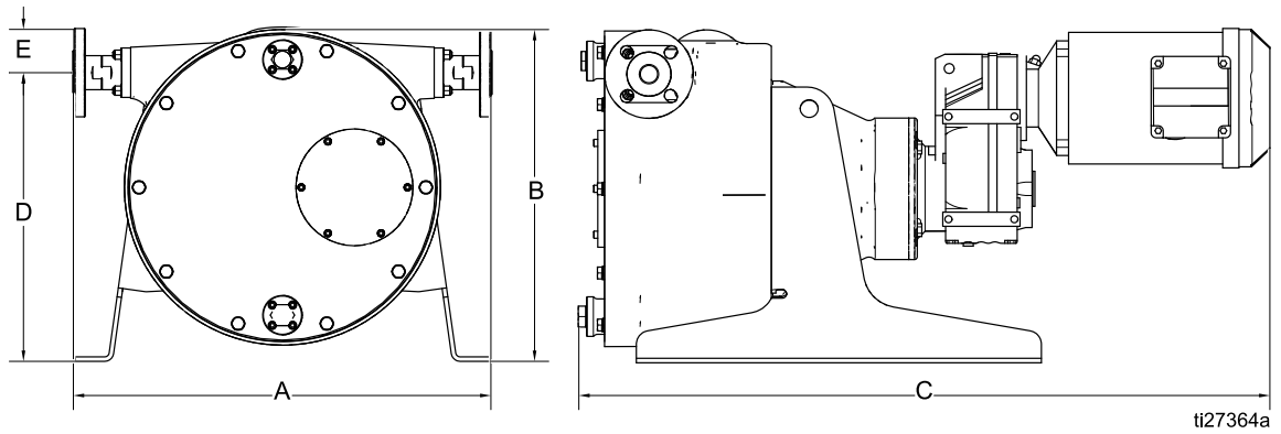
Figure 19 Wisselstroompompen ST26 en ST30
