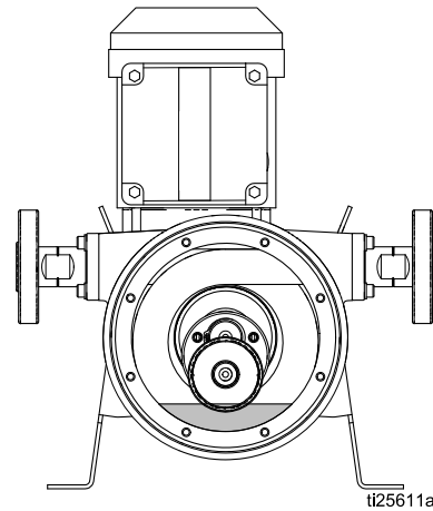
Figure 5 Smoermiddelniveau
