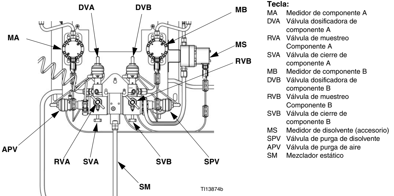
FIG. 10: Estación de fluido de montaje en muro, dosificación dinámica
