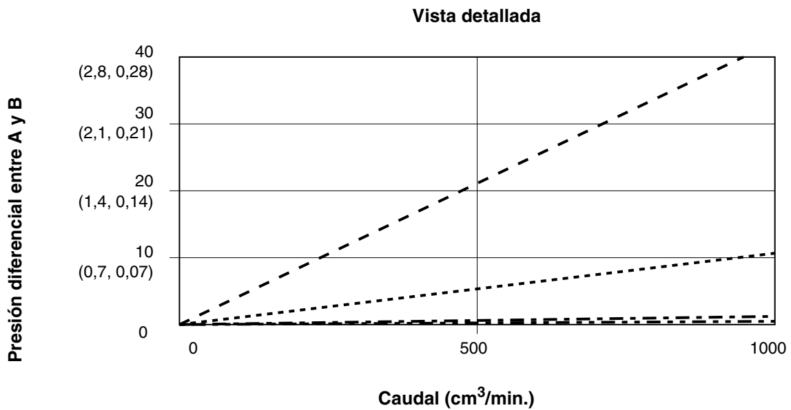
FIG. 23: Rendimiento de la dosificación dinámica (relación 30:1, fluido de 90 centipoises, presión de lado A 0,7 MPa [7 bar, 100 psi])
