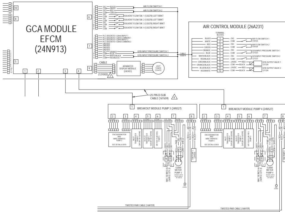
Figure 30 电气示意图，表 2，第 2 部分 下页续
