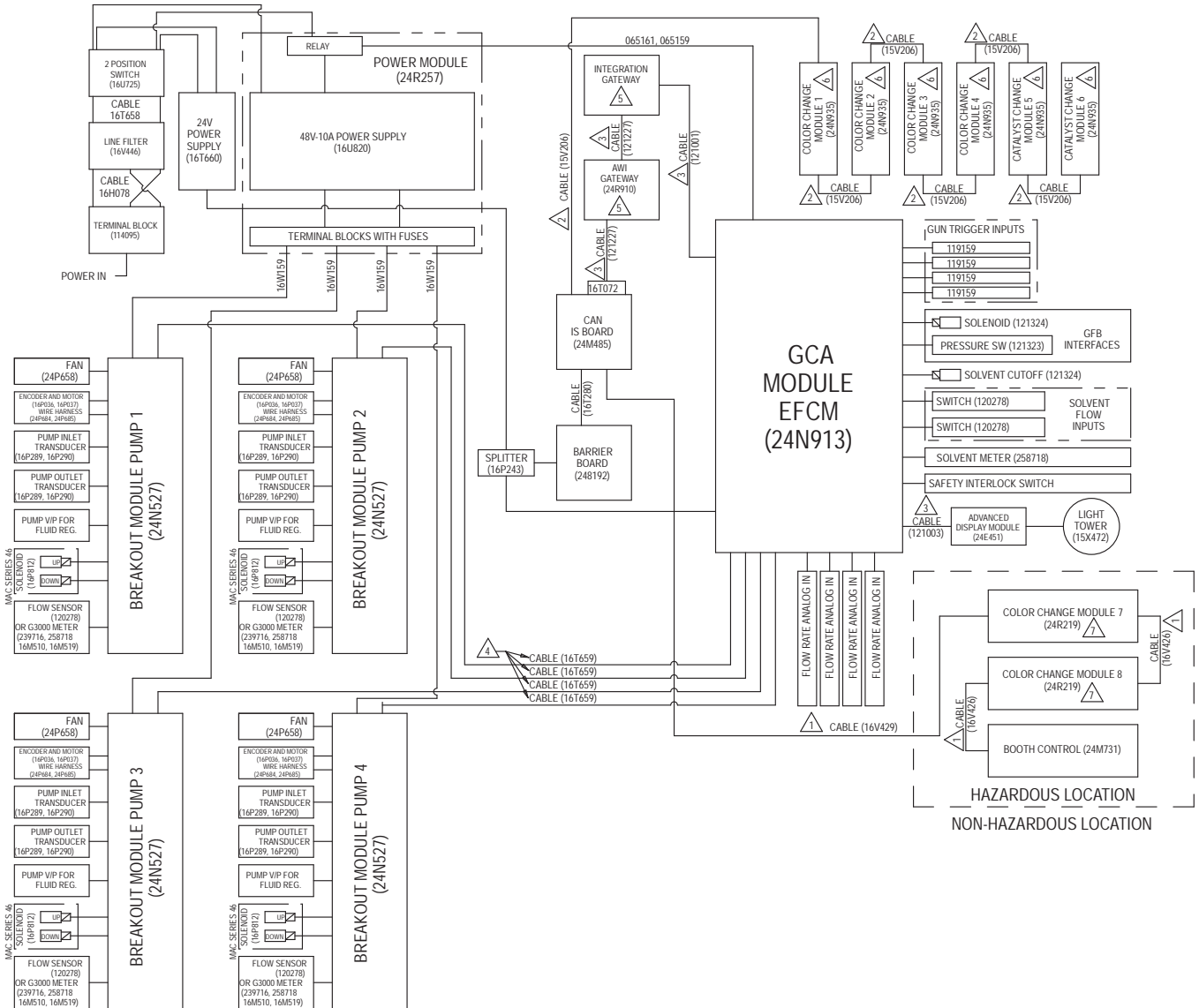
Figure 22 电气示意图, 表 1
