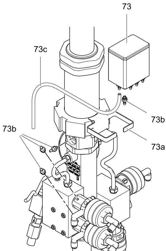
Figure 18 安装 TSL 杯套件
