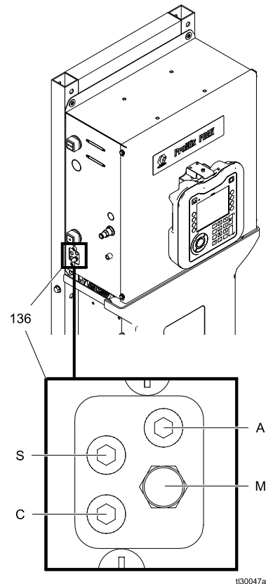
Figure 14 雾化空气和空气歧管连接图例
