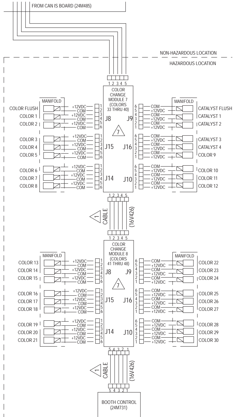
Figure 27 电气示意图，表 3，危险场所
