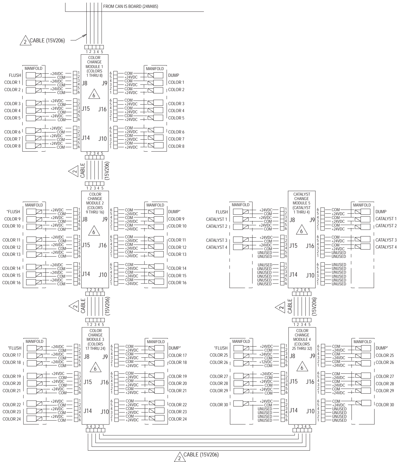
Figure 25 电气示意图，表 3
