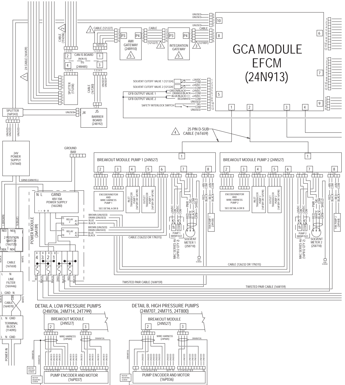
Figure 29 电气示意图，表 2，第 1 部分
