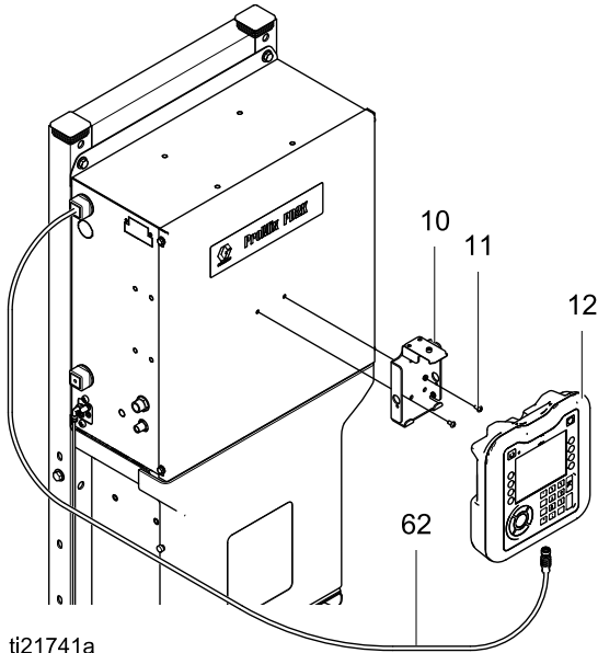
Figure 12 安装显示模块
