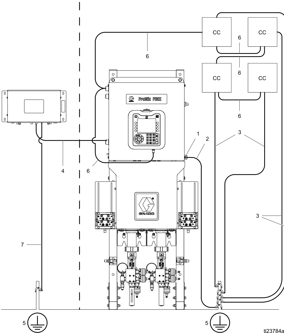
Figure 21 系统接地
