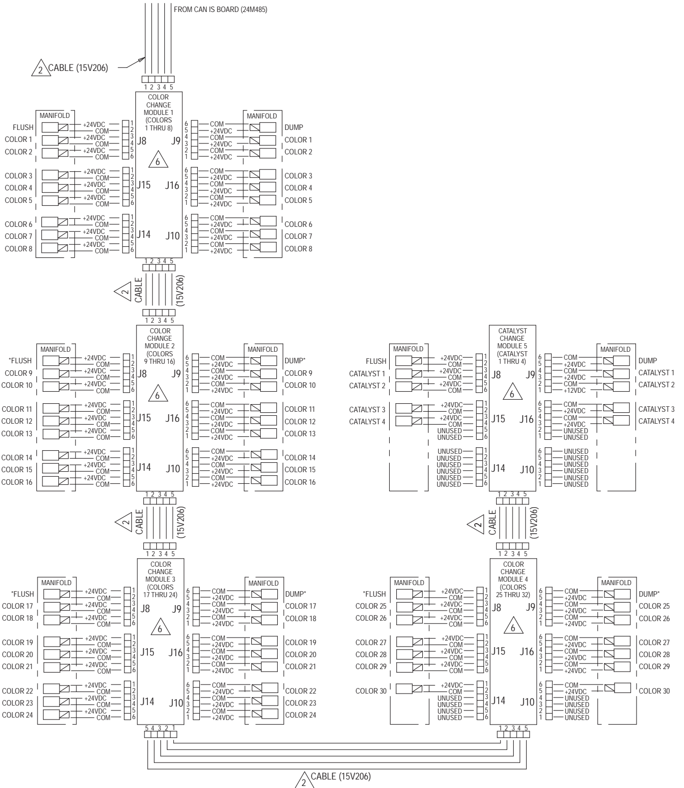
Figure 31 电气示意图，表 3，第 1 部分
