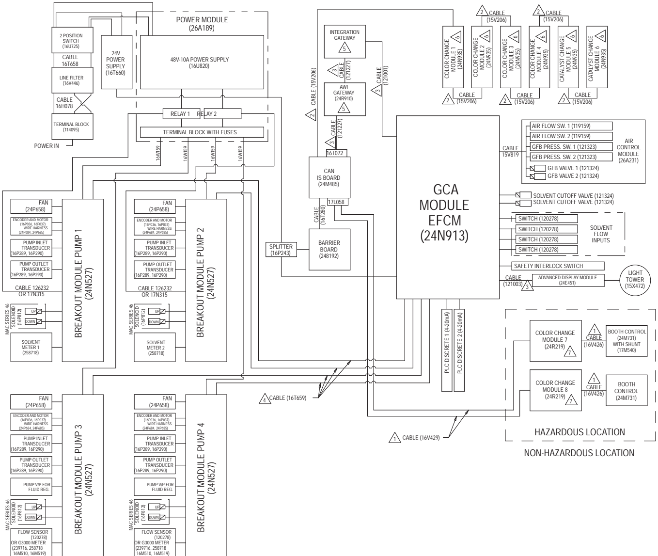
Figure 28 电气示意图，表 1
