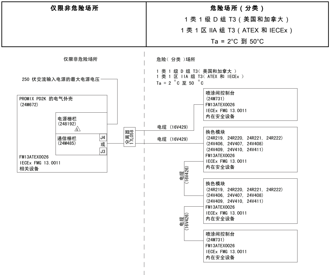
Figure 9 系统控制图 16P577
