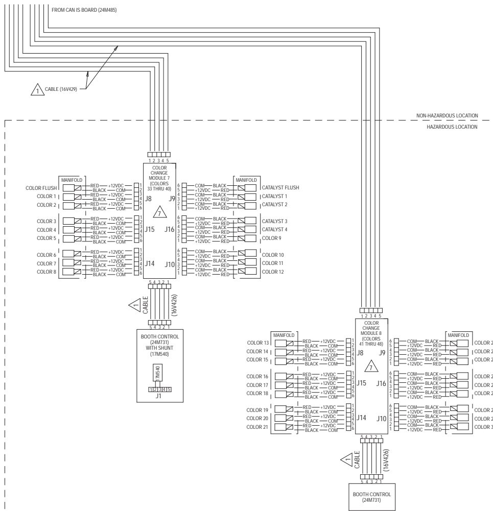
Figure 32 电气示意图，表 3，第 2 部分 下一页
