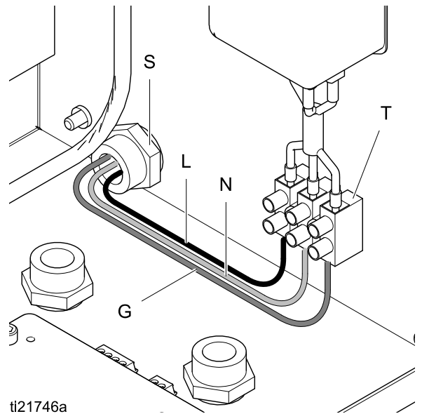
ti21746a Figure 19 控制箱电气连接
