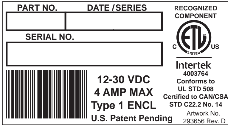
Figure 7 泵扩展套件 (附件) 识别标牌
