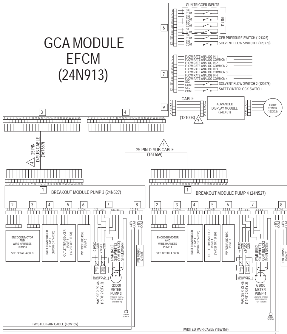
Figure 24 电气示意图, 表 2, 第 2 部分
