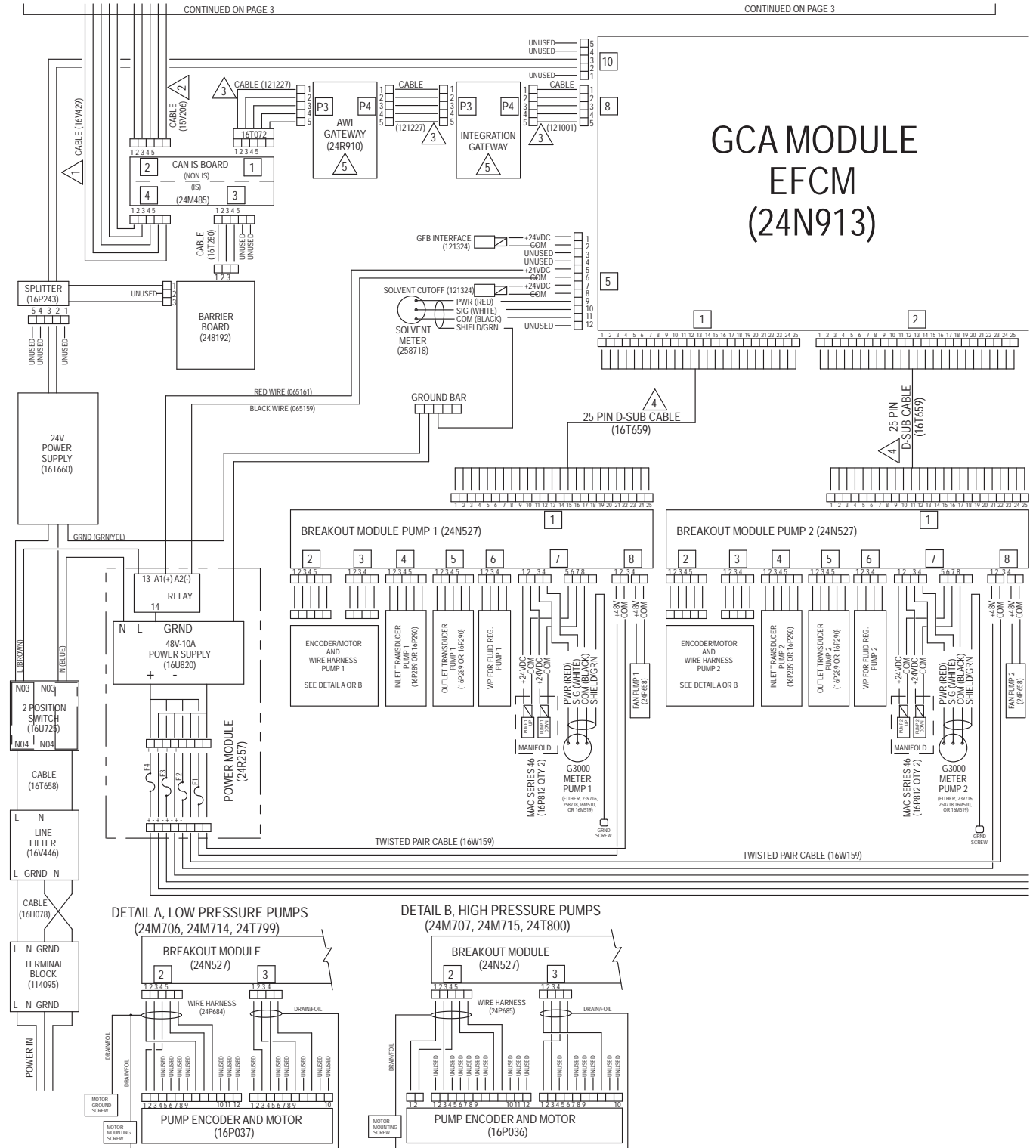
Figure 23 电气示意图，表 2，第 1 部分
