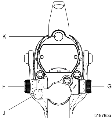
Figure 11 静电喷枪控制器
