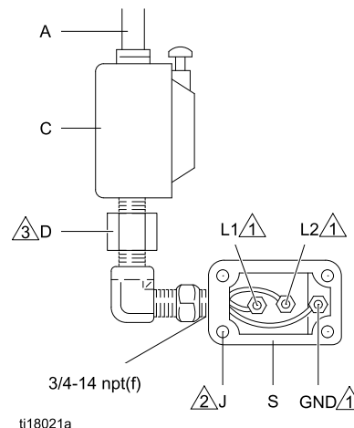
Figure 7 Conecte los cables de alimentación
