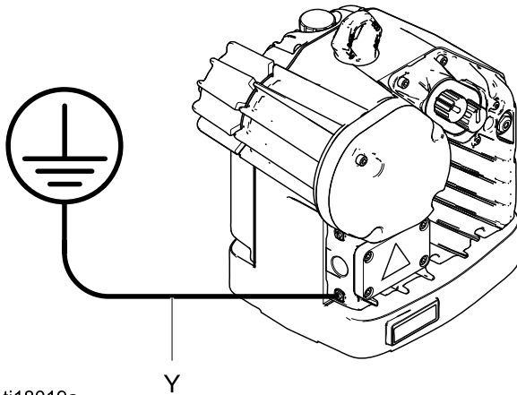
Figure 8 Cable de conexión de tierra
