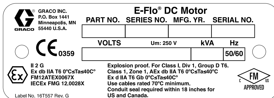
Figure 1 Etiqueta de identificación del motor básico
