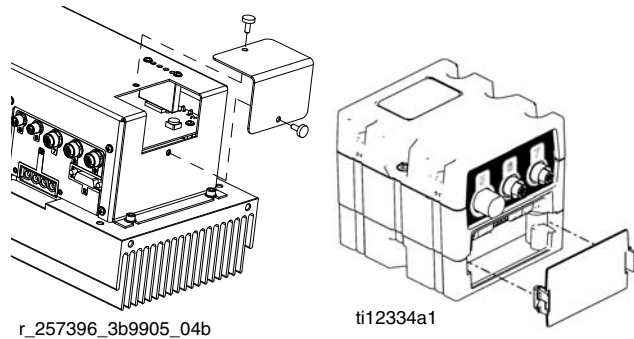
图 11: 移除检修盖
