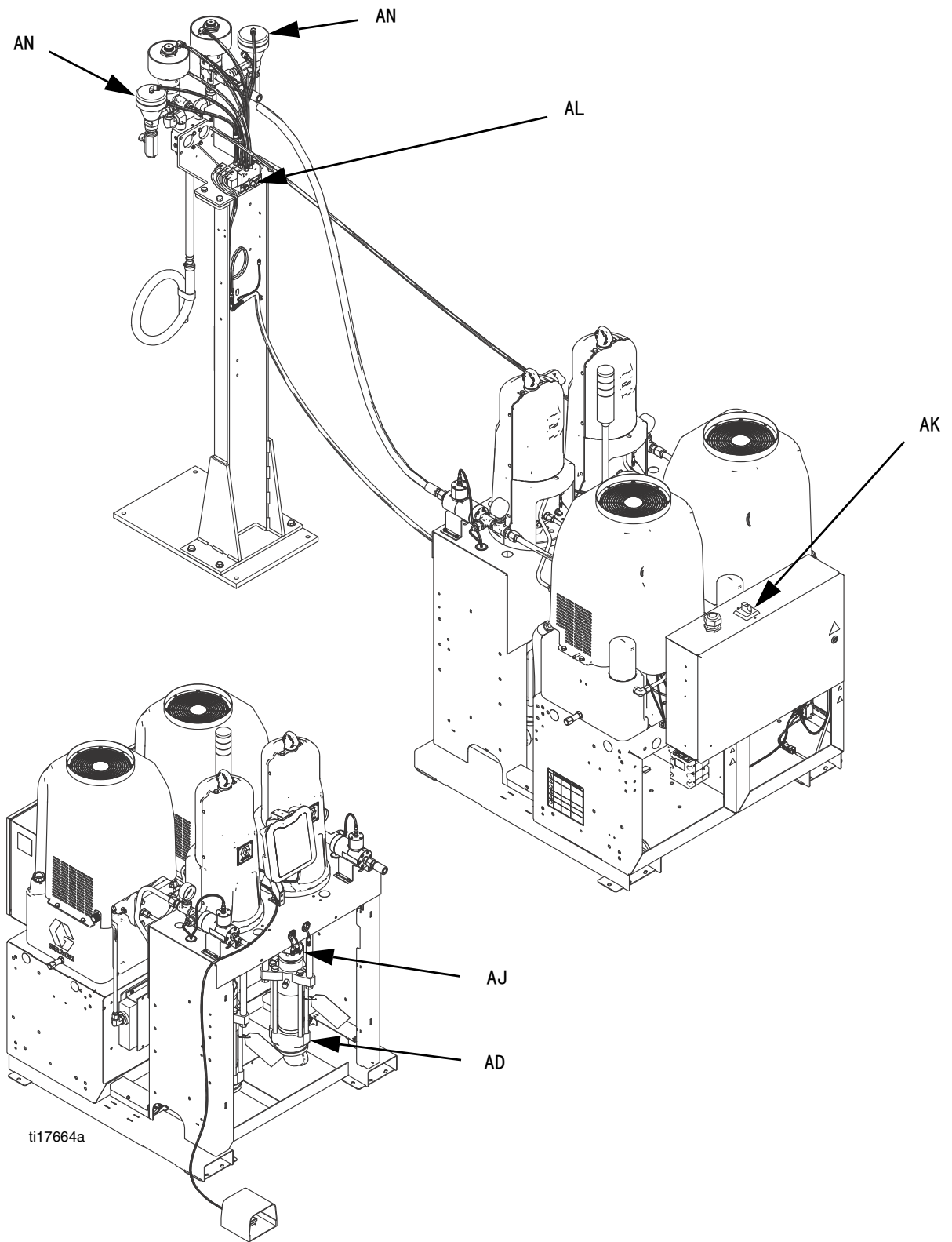
图 2：部件辨认
