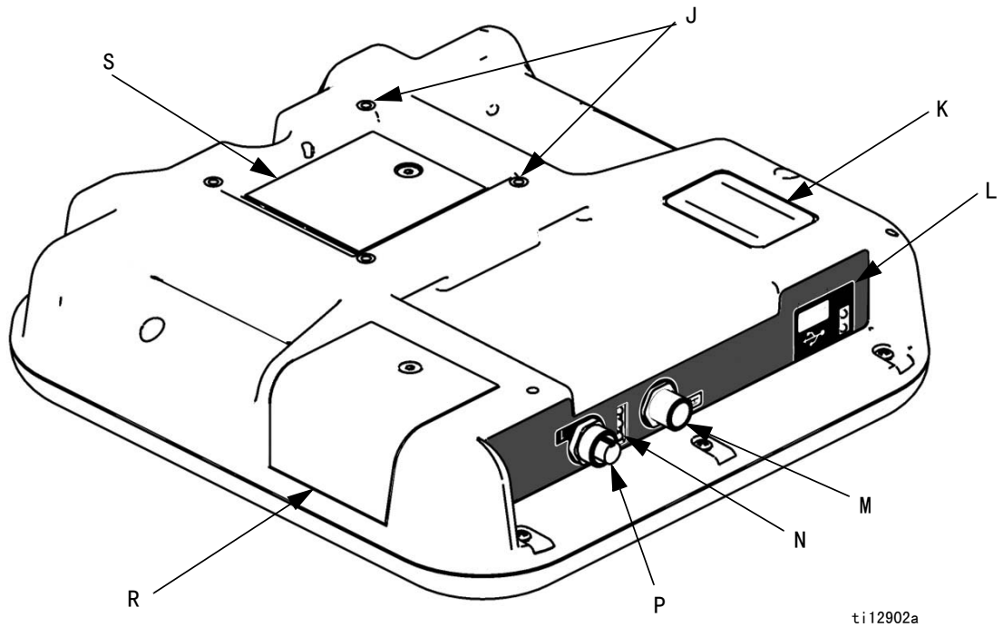
图 6: ADM 部件识别 - 后面
