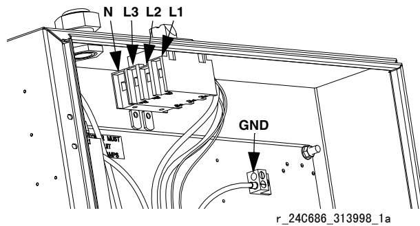
图 10：图示为 400V, 3 相
