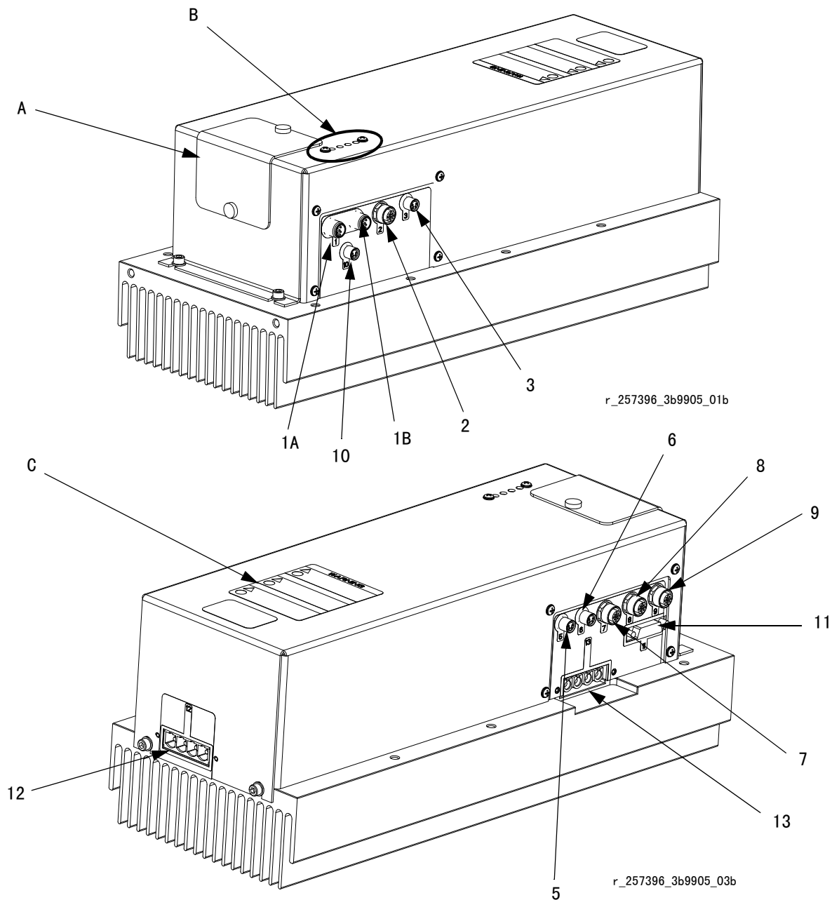
图 4: MCM 部件辨认
