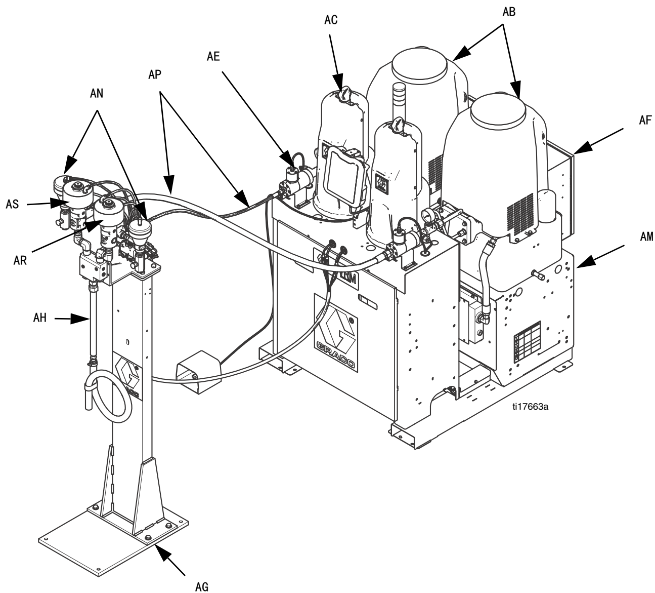
图 1: 部件辨认
