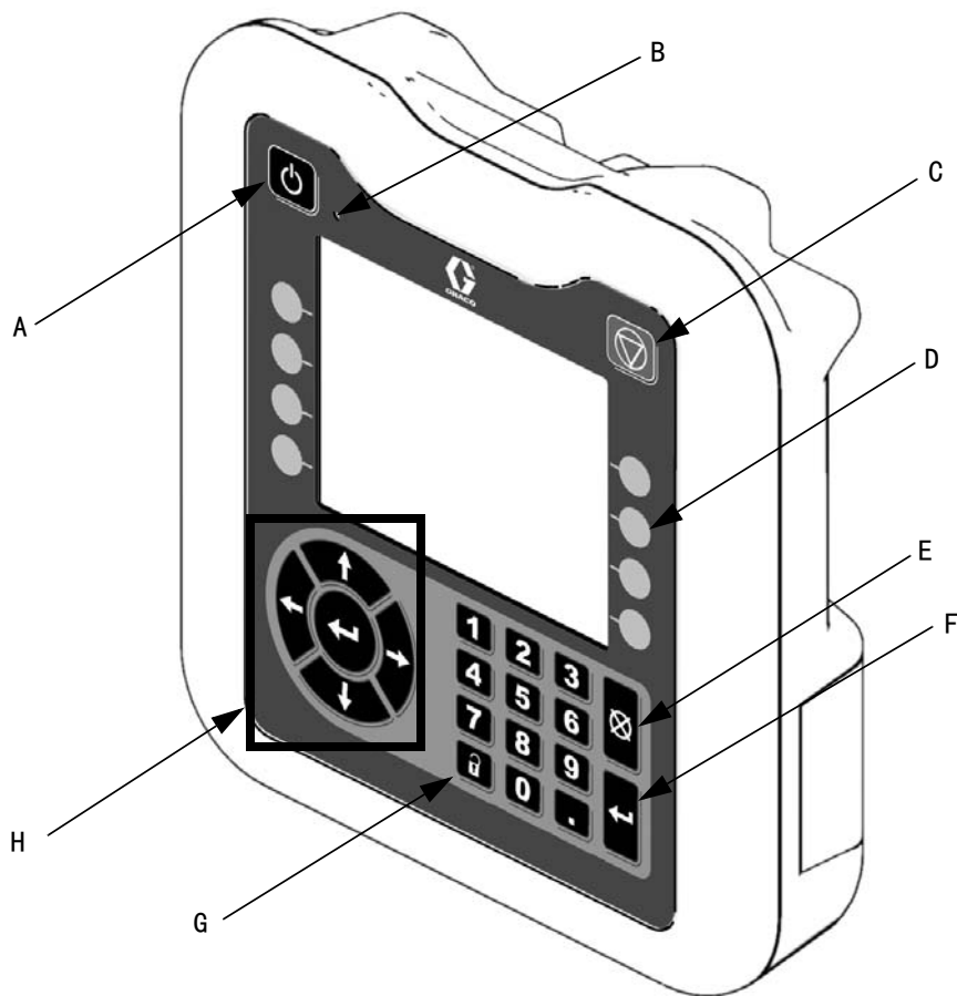
图 5: ADM 部件识别 - 前面
