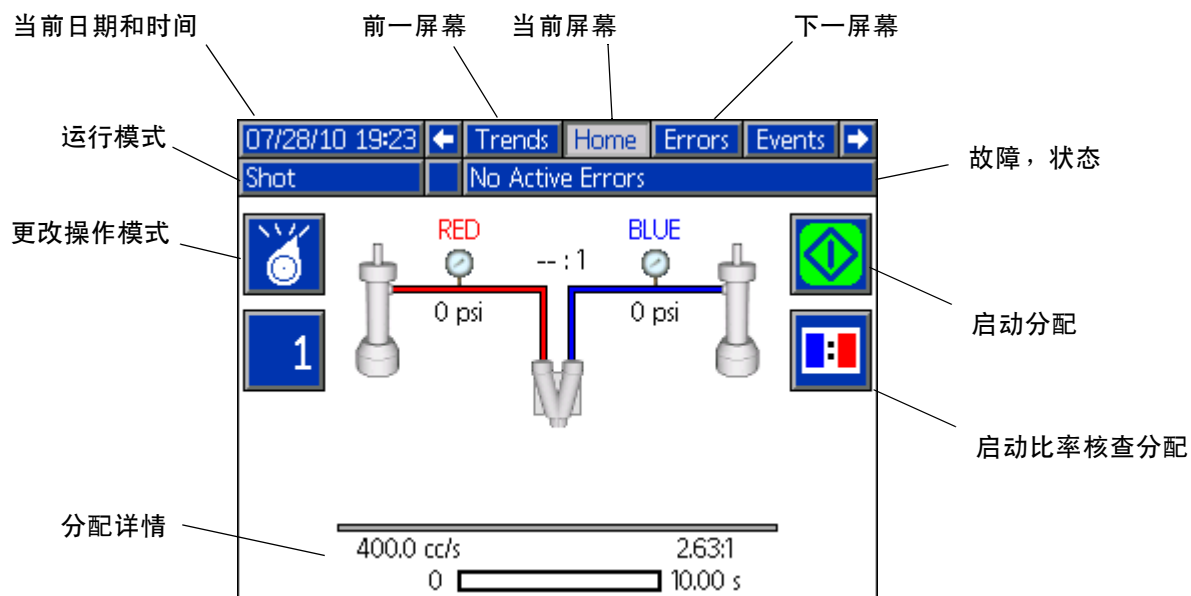
图 8: 主显示部件 - 主屏幕 ( 图示为喷射模式 )
