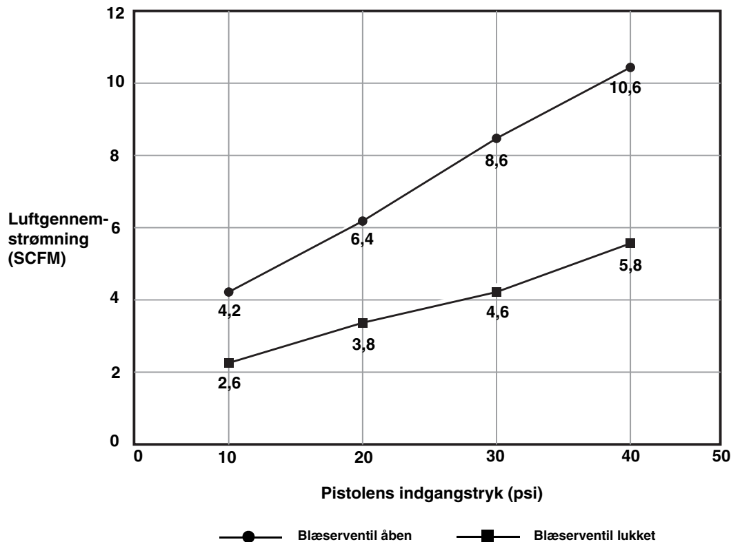
Luftgennemstrømning, standardlufthætte, serie AA
