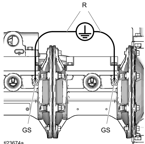
Figure 1 Vis et fils de terre
