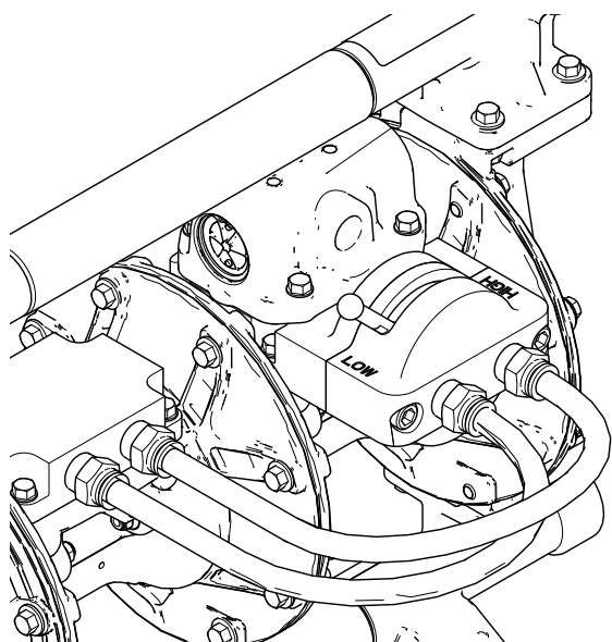
Figure 4 Levier de basse/haute pression
