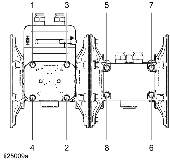
Fixations de la vanne d'air
