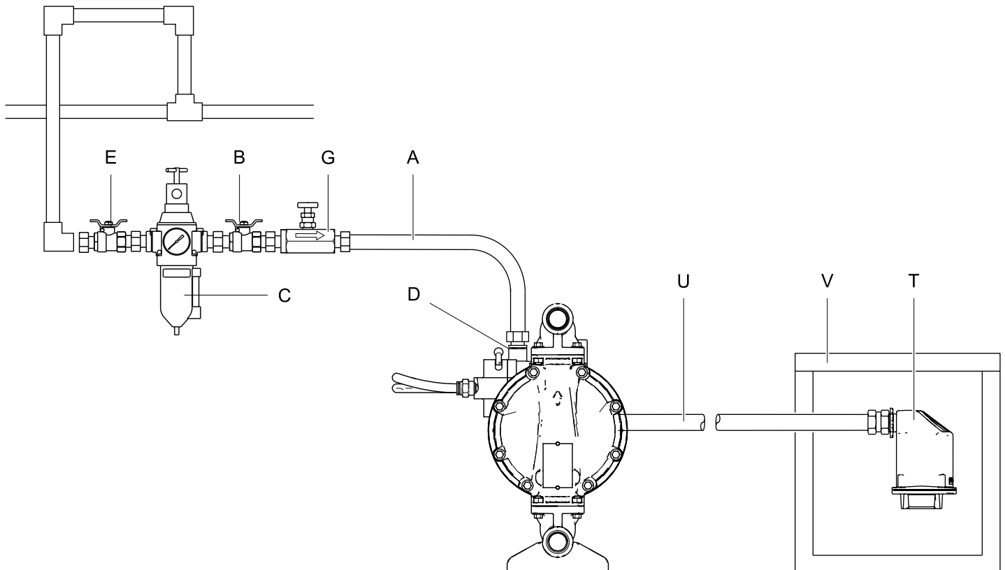
Figure 2 Ventilation de l'air d'échappement
