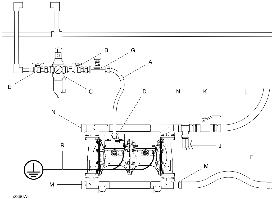
Figure 3 Installation normale avec montage au sol
