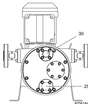
Figure 1 Aftapgat (29) en ontluichtingsgat (30) van de pomp
