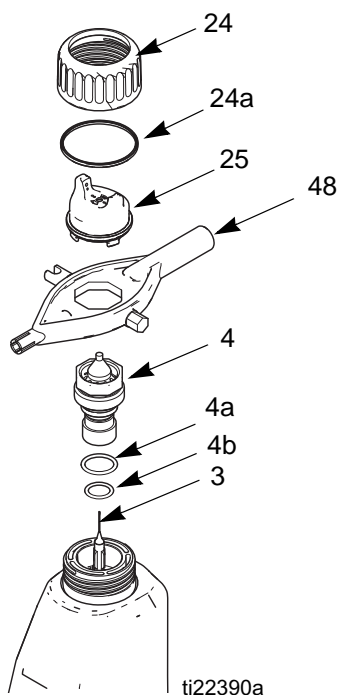
FIG. 18. Luftkappe/Düse ersetzen
