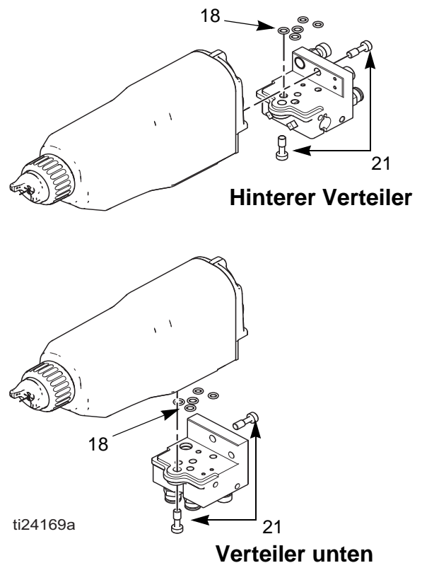
Fig. 17. Pistole vom Verteiler abnehmen
