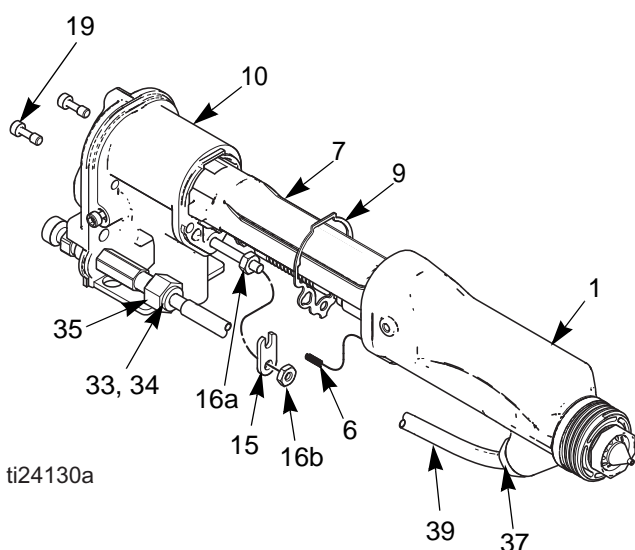
FIG. 25. Einbau des Laufs
