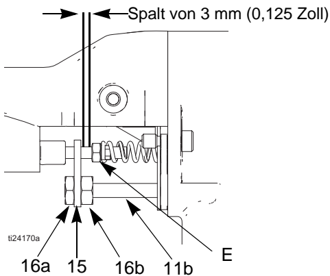
FIG. 23. Stellgliedeinstellung
