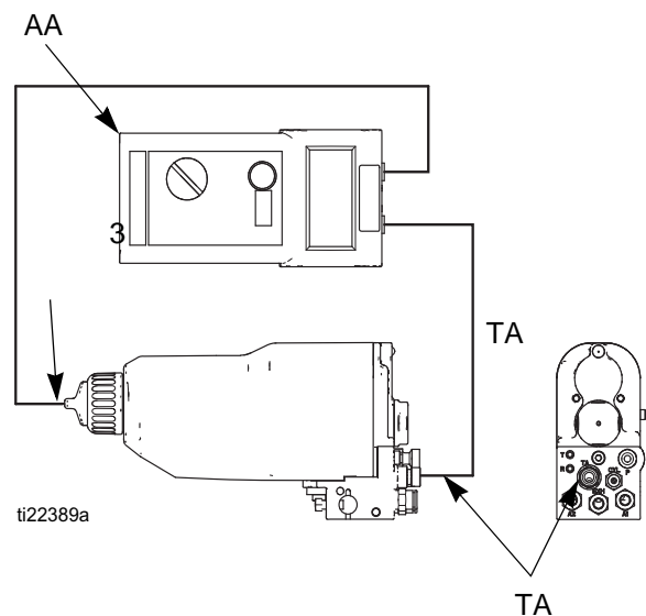
FIG. 14. Pistolenwiderstand überprüfen
