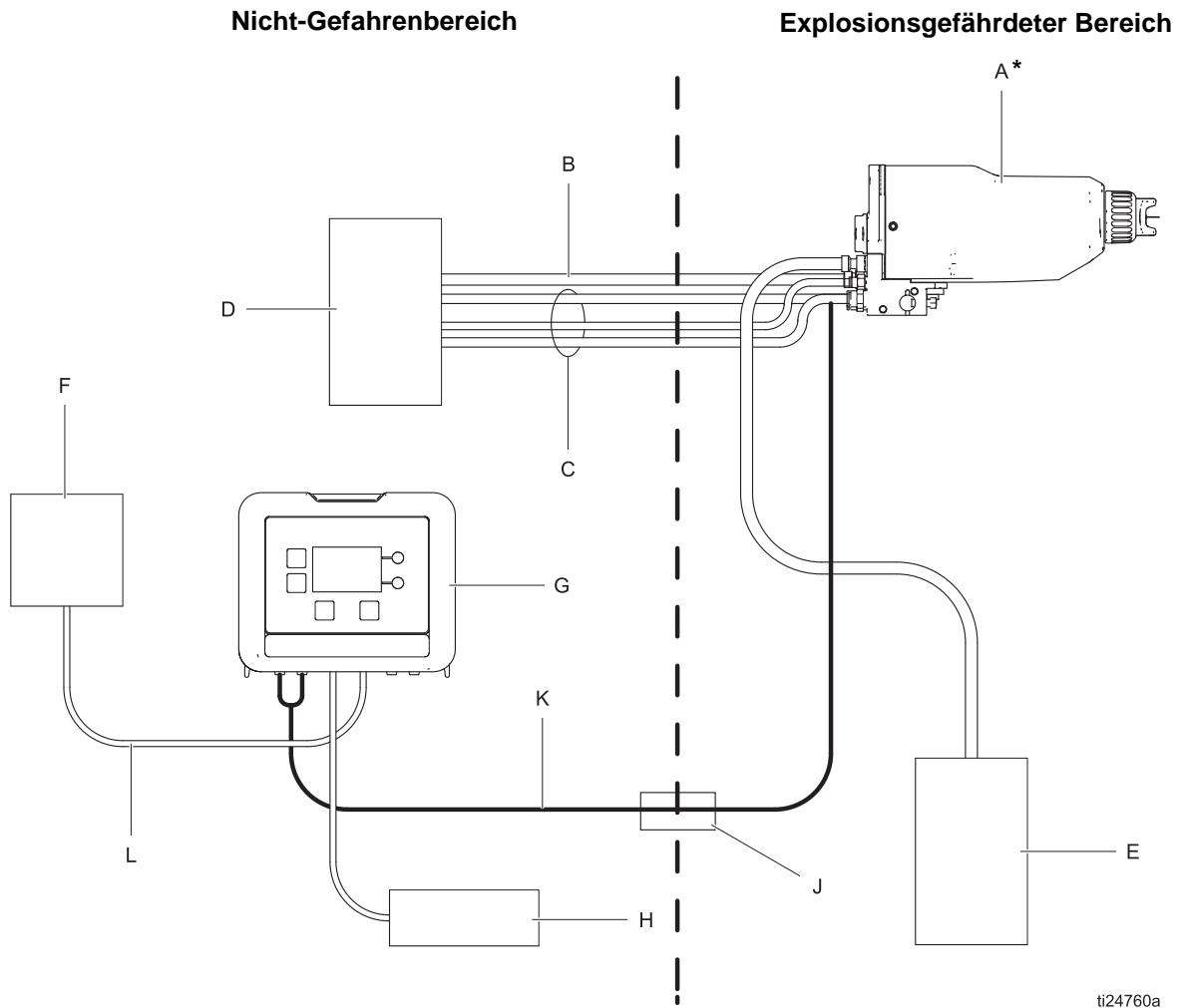
FIG. 1. Typische Systeminstallation
