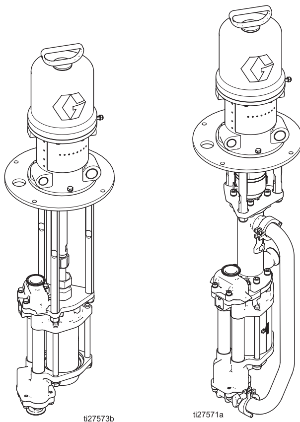
Pompa President con unità pompante a 4 sfere sigillata
