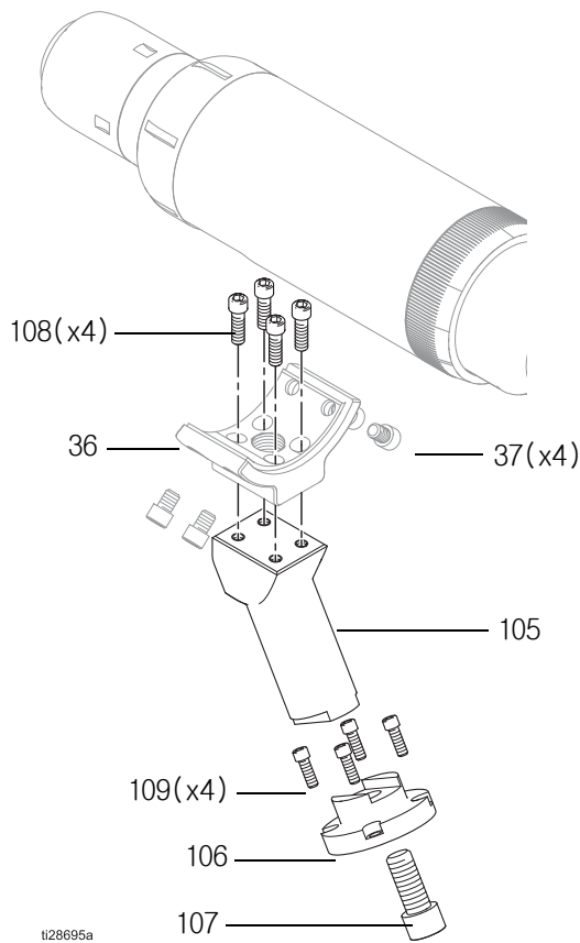
그림 4 60° 로봇 장착
