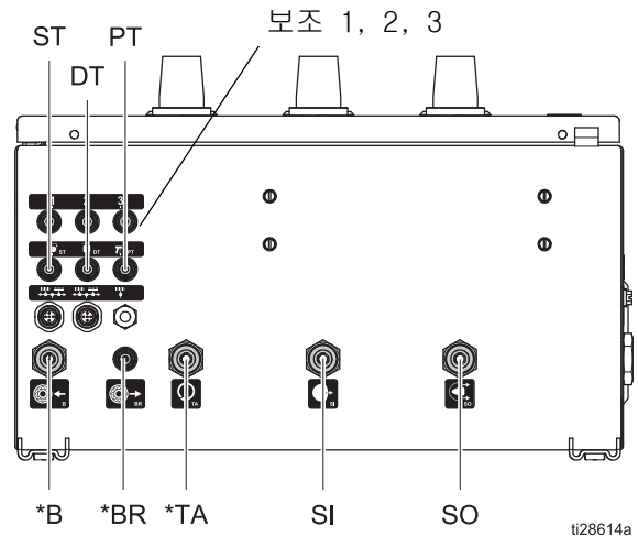
그림 15. 에어 연결, 수동 에어 컨트롤러
