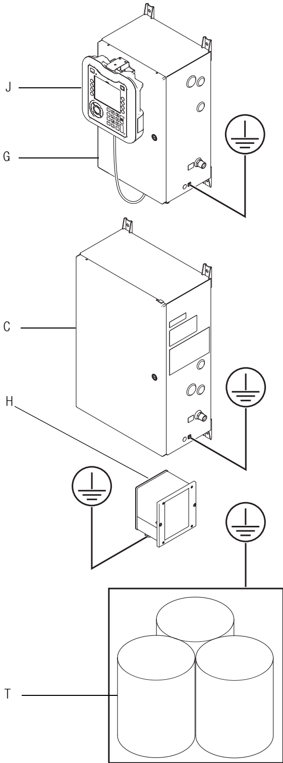
그림 17. 시스템 접지
