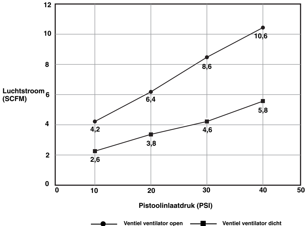
Luchtstroom, standaard AA serie luchtkap
