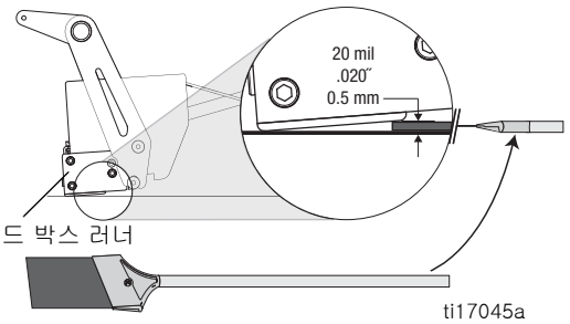
스크리드 박스
