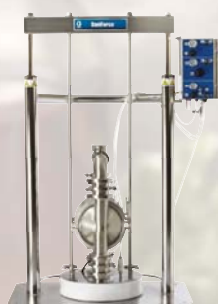
SaniForce 3150 HS Dépoteur de fût
