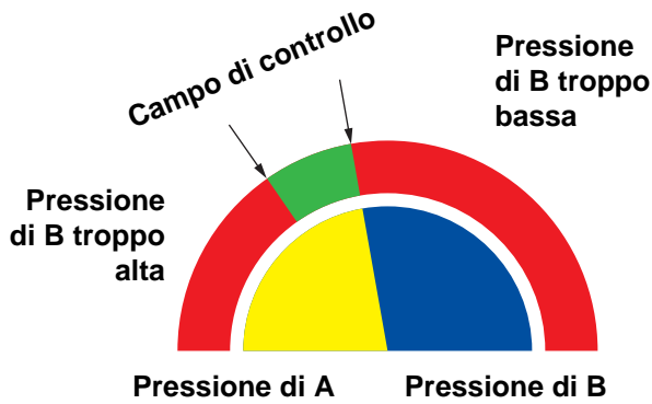
FIG. 50. Campo di controllo A/B con ugello di strozzamento di dimensioni corrette
