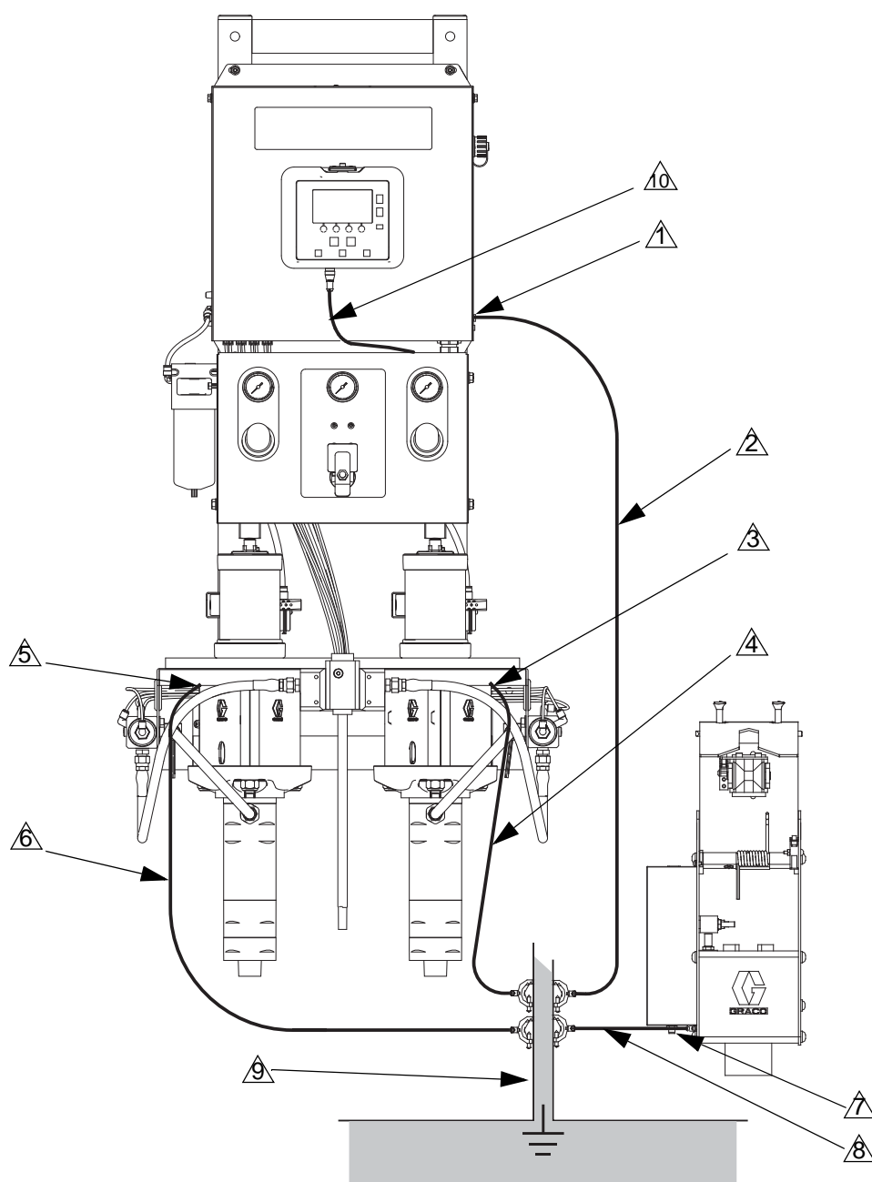
FIG. 9. Messa a terra
