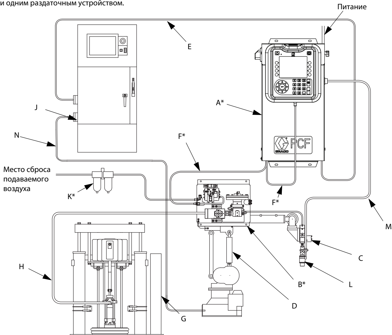
Рис. 1: Стандартная конфигурация системы, работающей при температуре окружающей среды
