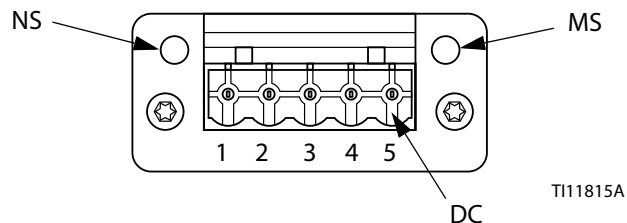
Рис. 74: Соединения промышленной сети DeviceNet
