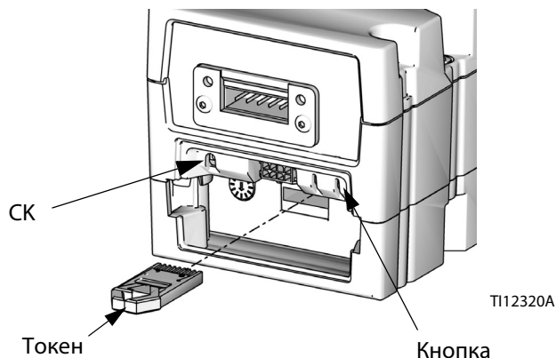
Рис. 49: Вставка токена
