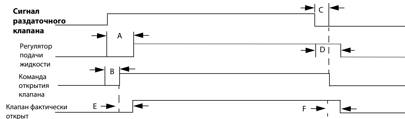
Рис. 32: Задержка срабатывания
