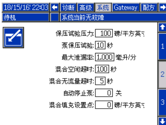
Figure 30 系统屏幕 2 处于待机模式
