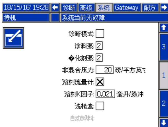
Figure 28 系统屏幕 1，待机期间
