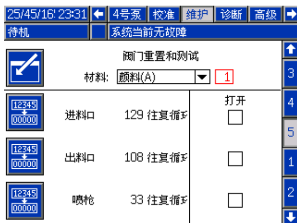
Figure 58 维护屏幕 4，颜色阀重置
