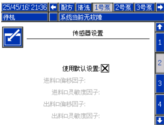
Figure 44 泵屏幕 2，默认设置已启用
