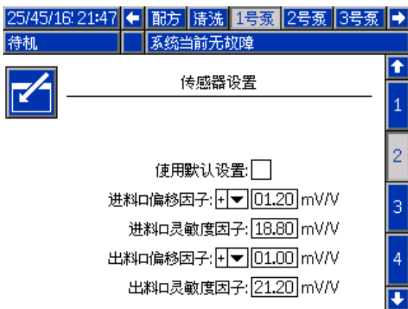
Figure 45 泵屏幕 2，默认设置已禁用
