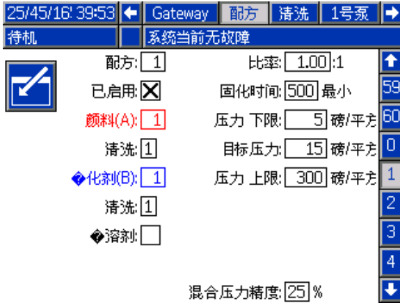
Figure 39 有效配方屏幕
