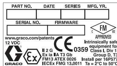
Figure 5 内在安全性换色控制 ( 附件 ) 标识标牌
