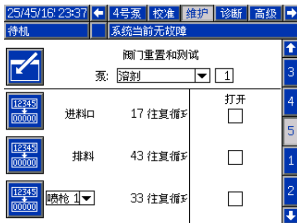
Figure 59 维护屏幕 4，溶剂阀重置
