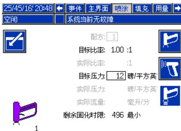
Figure 18 喷涂屏幕，处于空闲模式
