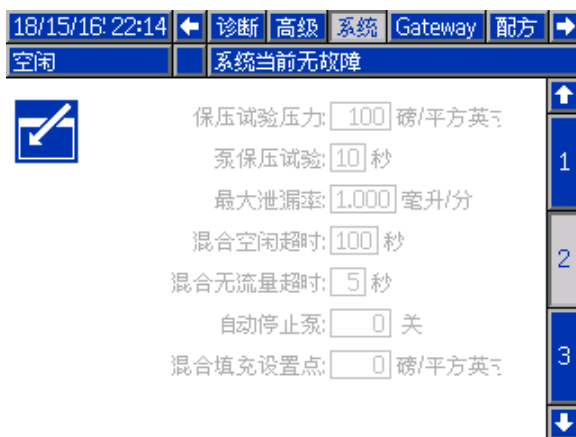
Figure 31 系统屏幕 2，处于混合模式
