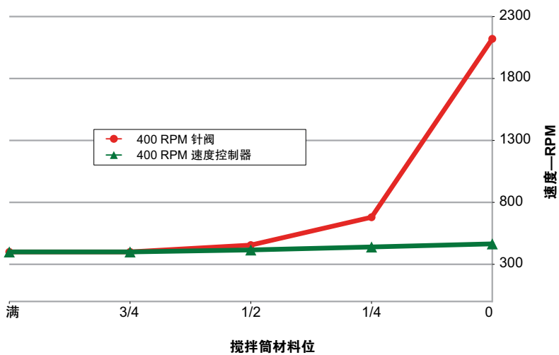
速度控制器和针阀比较
