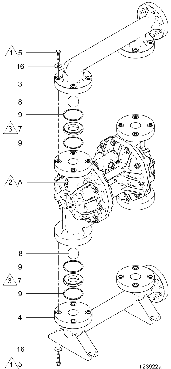
Figure 1 チェックバルブアセンブリ
