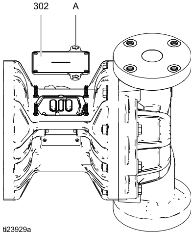
Figure 2 液体カバーツール
