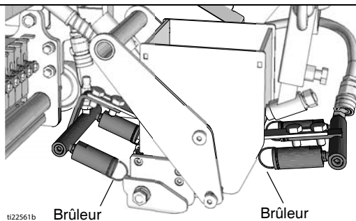
FlexDie Brûleurs (ThermoLazer 200/200TC)
