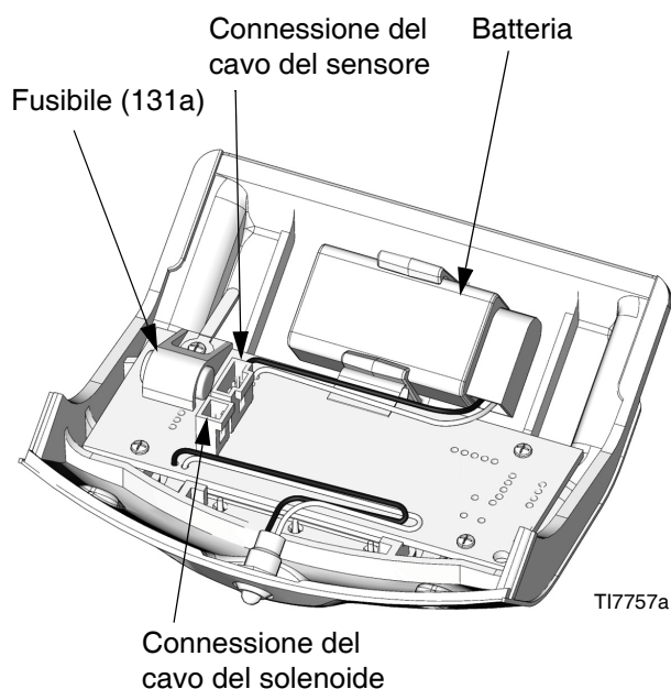
FIG. 5. Posizione del fusibile e della batteria del DataTrak
