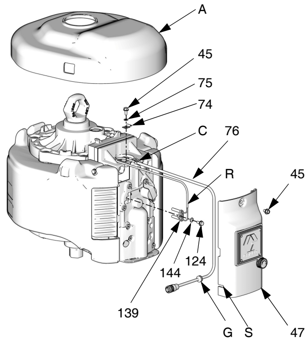
FIG. 17. Kit di collegamento per DataTrak remoto
