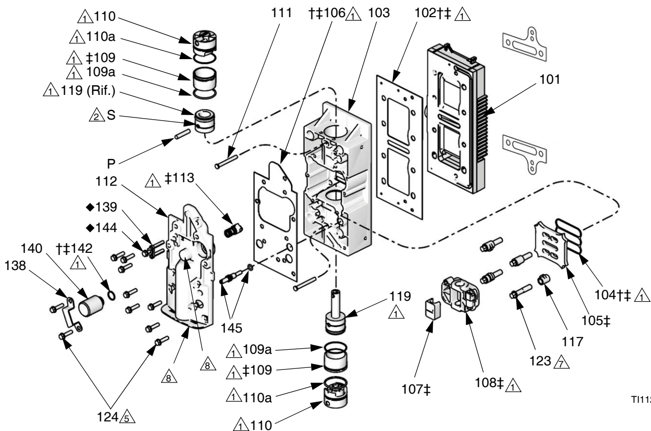
FIG. 11. Riparazione della valvola dell'aria (illustrato NXT107)
