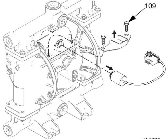
FIG. 2. Extracción del solenoide
