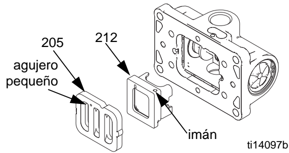
FIG. 6. Instalación de la copela y de la placa de la válvula de aire
