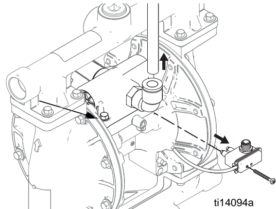
FIG. 1. Conjunto del interruptor de lengüeta y extracción de la línea de aire
