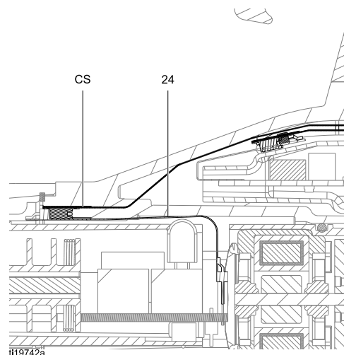
Figure 26 连接柔性电路
