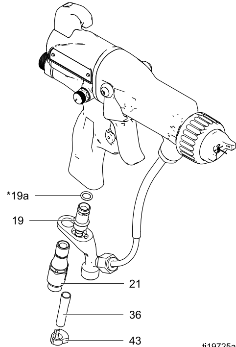
Figure 40 空气入口管接头和排气阀
