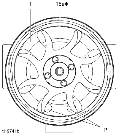
Figure 28 风扇方向
