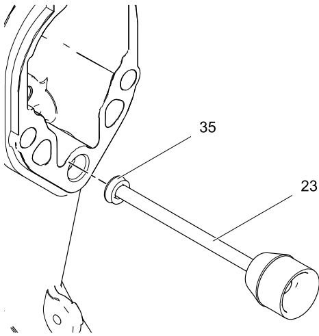
Figure 36 安装 U 形杯
