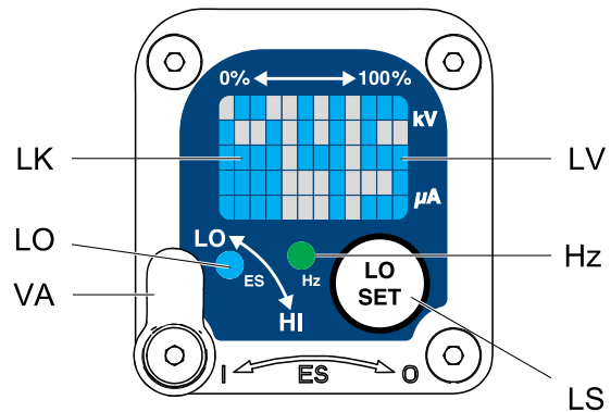
ti19337a Figure 5 低压设置屏幕 (已锁定)。
