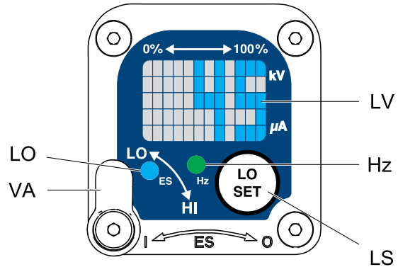
ti19122a Figure 4 低压设置屏幕 (未锁定)
