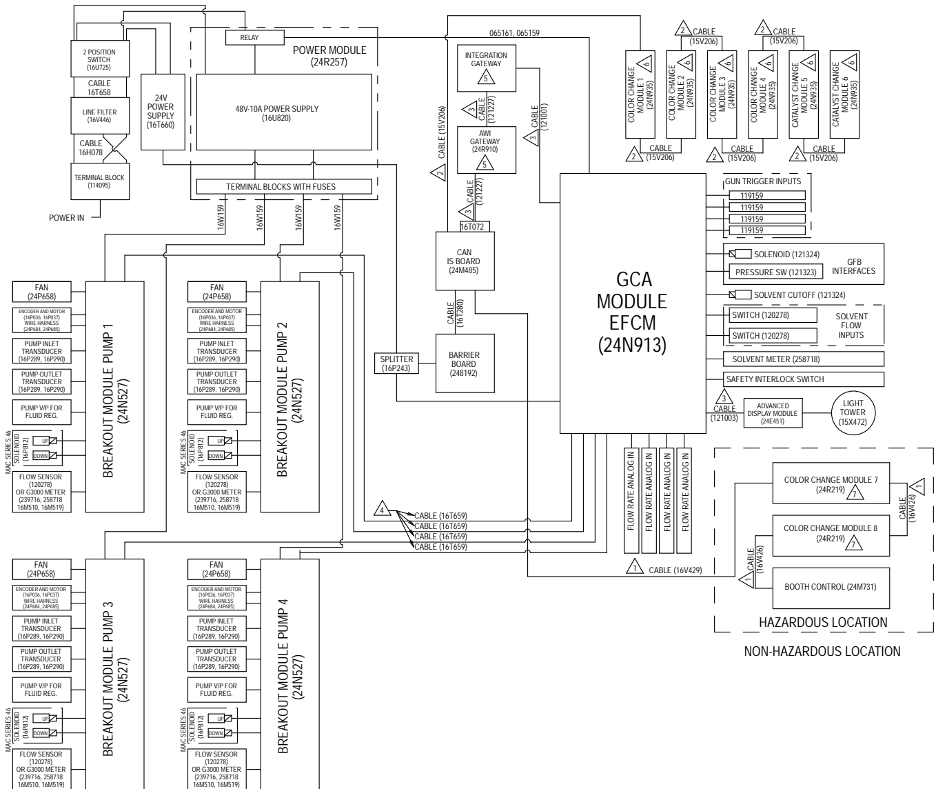
Figure 24 Электросхема, лист 1
