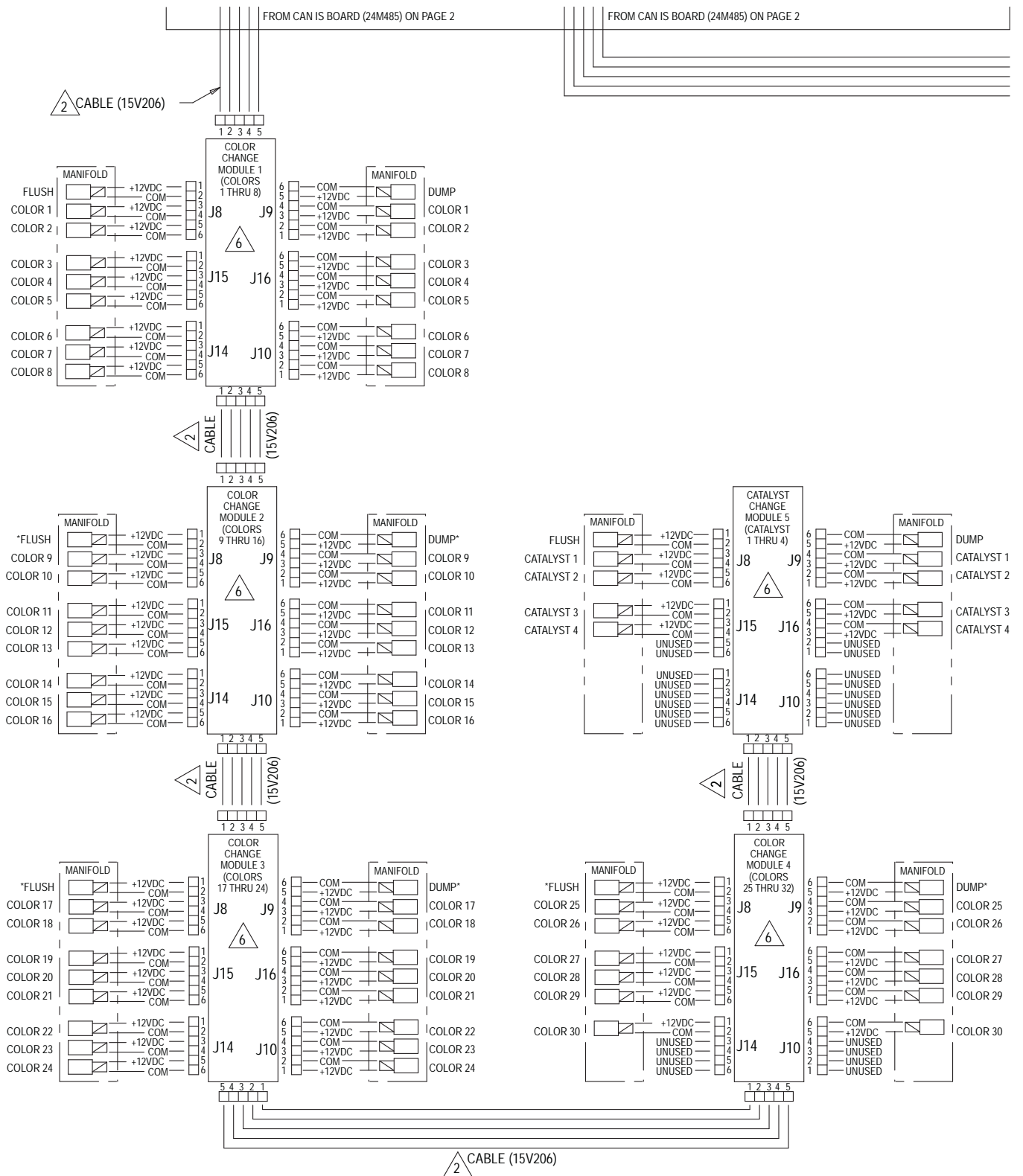
Figure 27 Электросхема, лист 3
