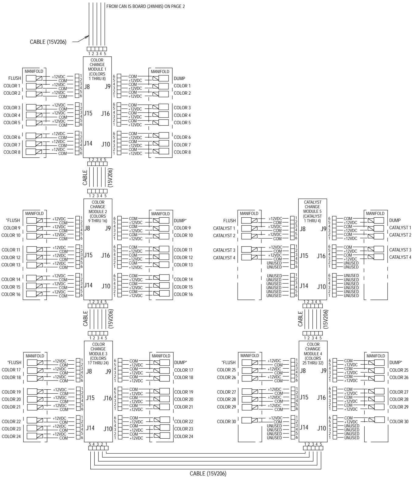
Figure 33 Электросхема, лист 3, часть 1
