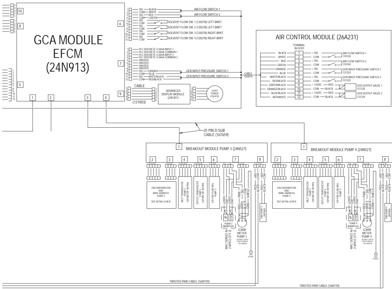
Figure 32 Электросхема, лист 2, часть 2 ПРОДОЛЖЕНИЕ НА СЛЕДУЮЩЕЙ СТРАНИЦЕ
