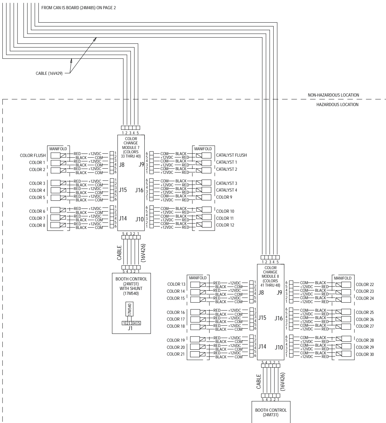
Figure 34 Электросхема, лист 3, часть 2 ПРОДОЛЖЕНИЕ НА СЛЕДУЮЩЕЙ СТРАНИЦЕ
