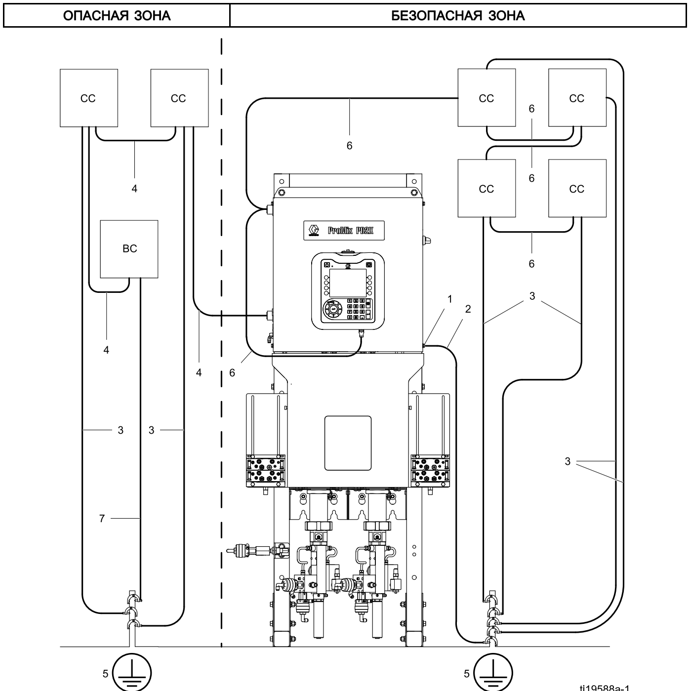
Figure 23 Заземление системы
