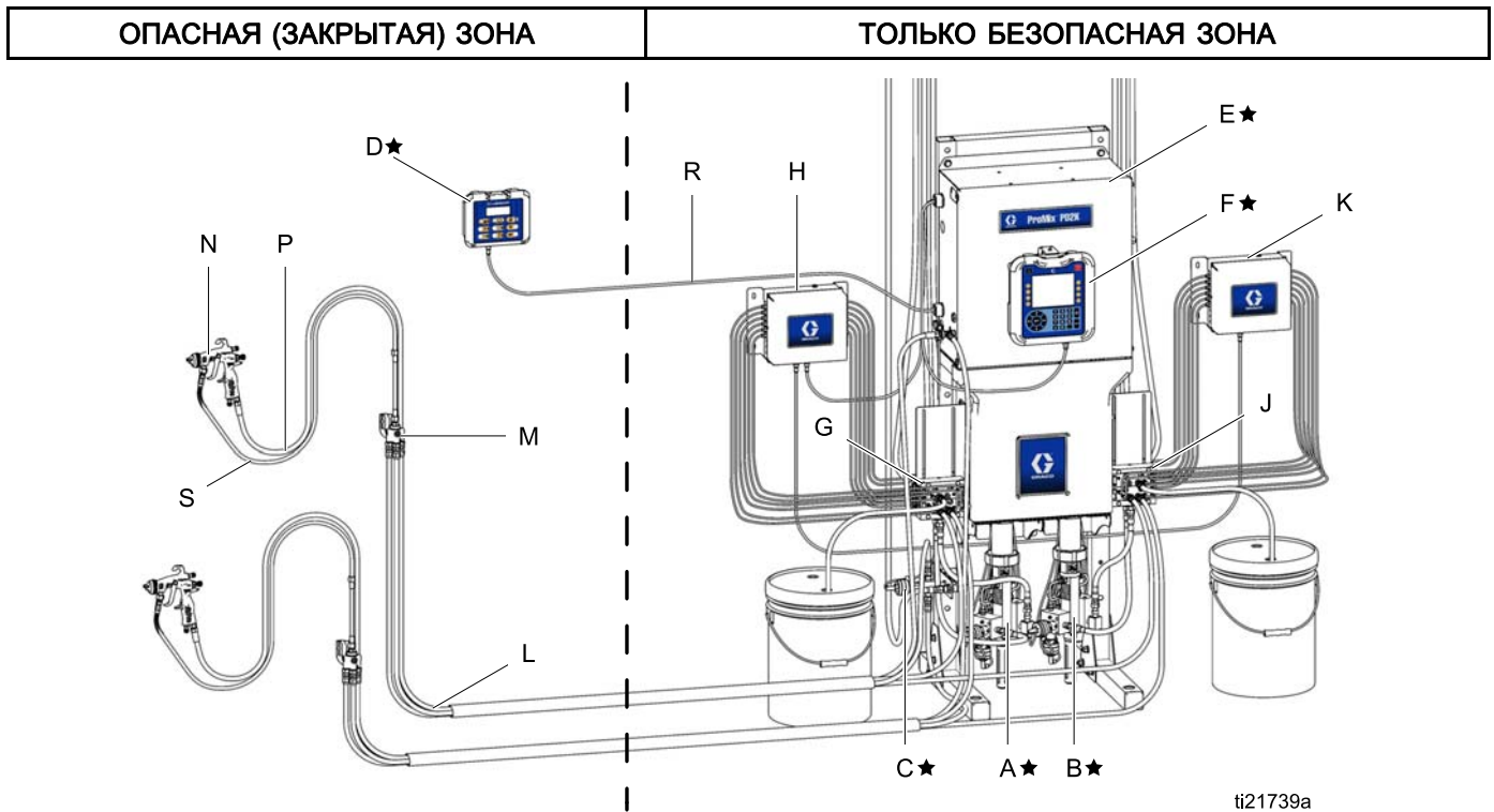
Figure 9 Типовая установка
