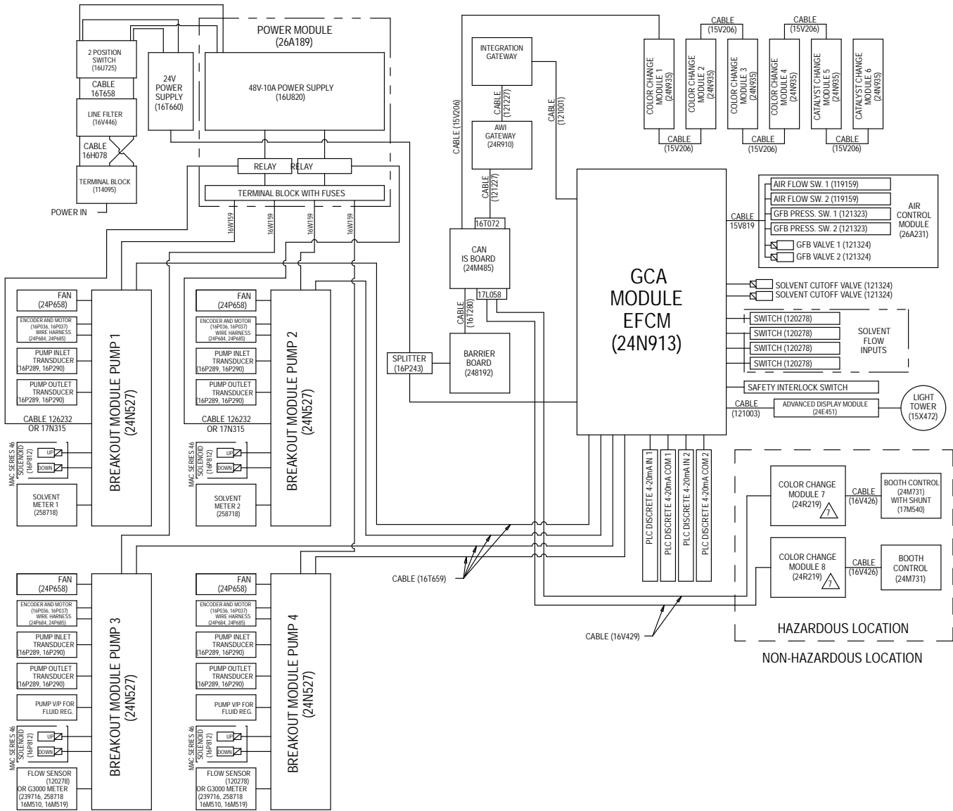
Figure 30 Электросхема, лист 1
