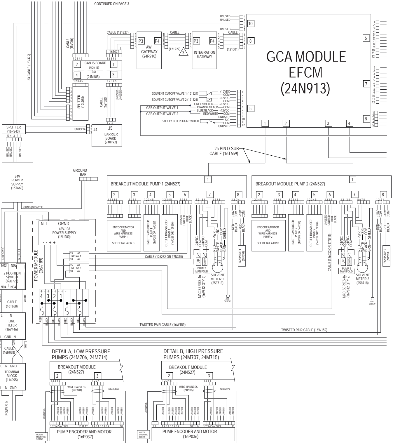
Figure 31 Электросхема, лист 2, часть 1 ПРОДОЛЖЕНИЕ НА СЛЕДУЮЩЕЙ СТРАНИЦЕ
