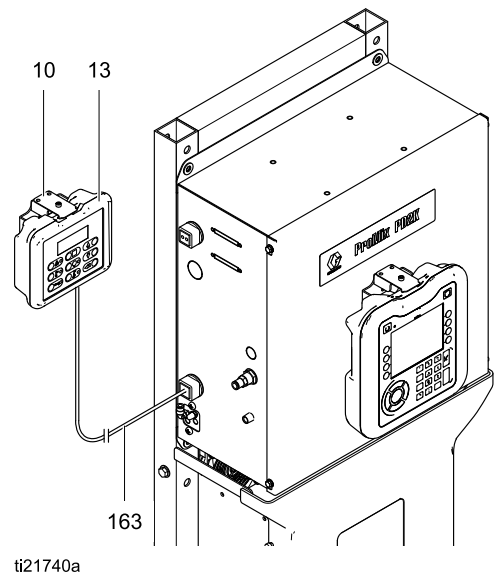
Figure 15 Установка устройства управления окрасочной камерой
