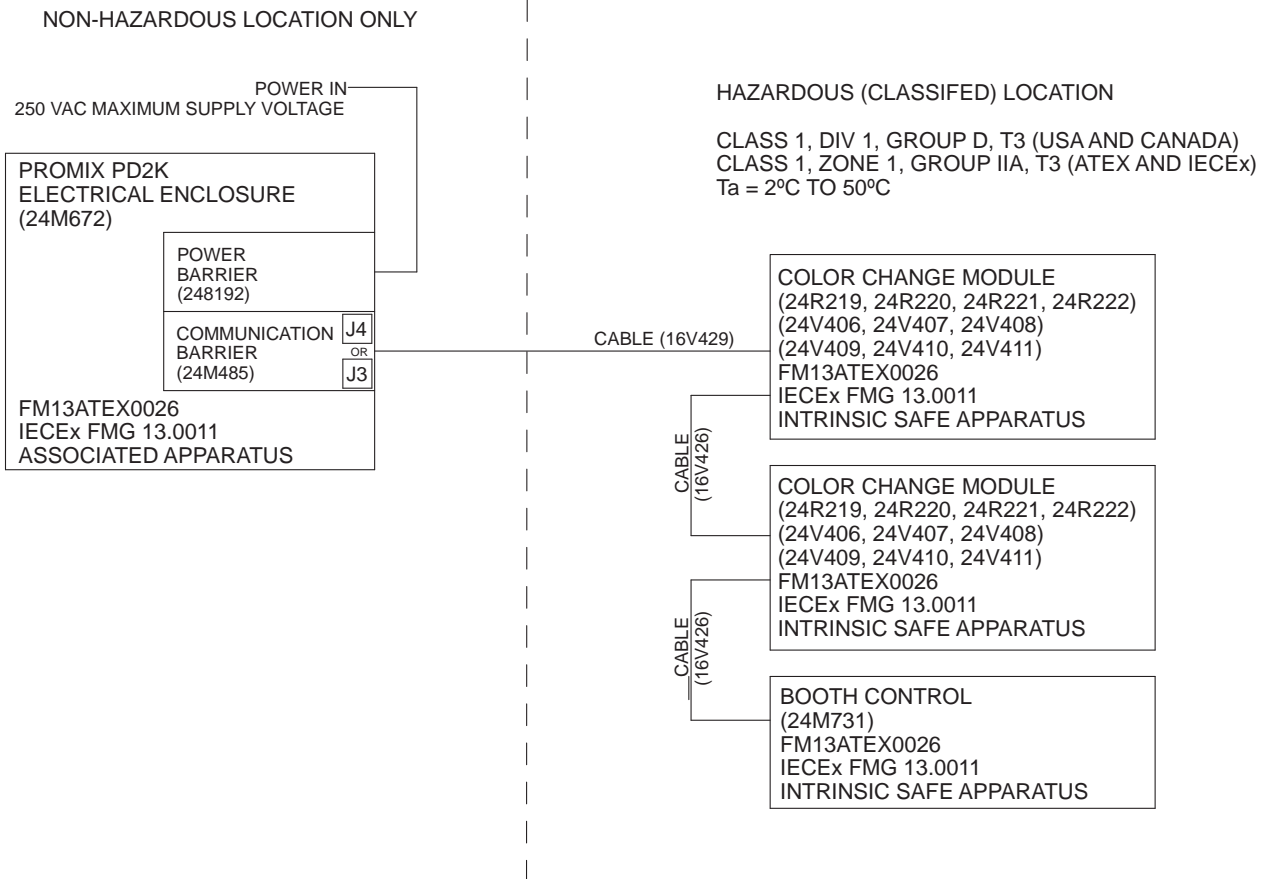
Figure 8 Контрольная схема системы 16P577
