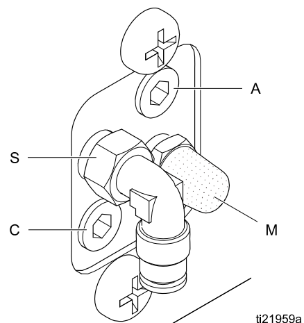
Figure 17 Соединения воздушного коллектора Обозначения
