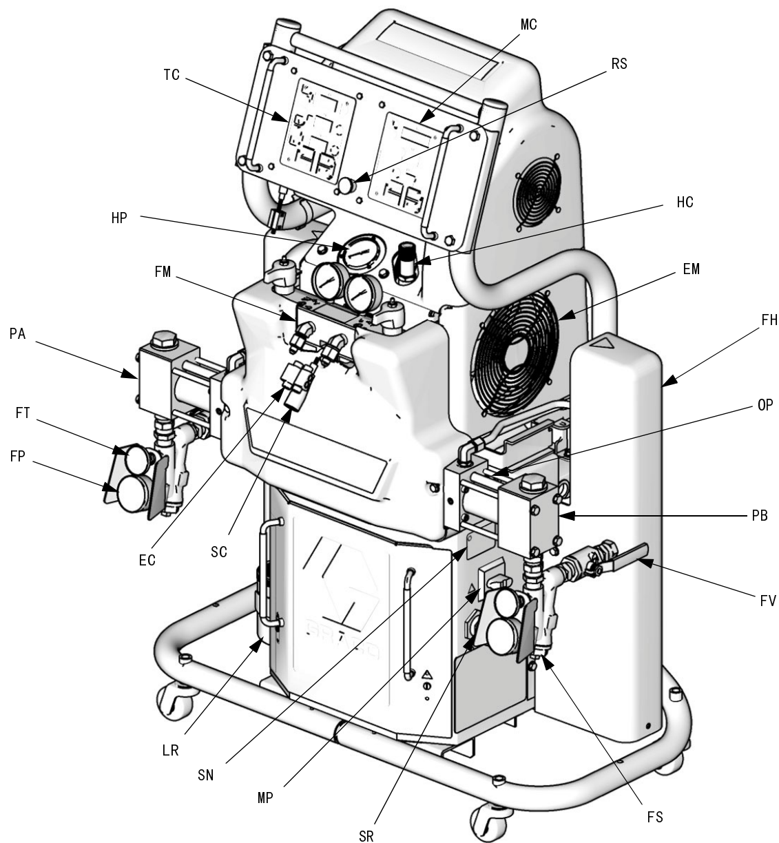
Reactor 流体歧管 ( 为便于清楚说明, 已取下护罩 ) 详图
