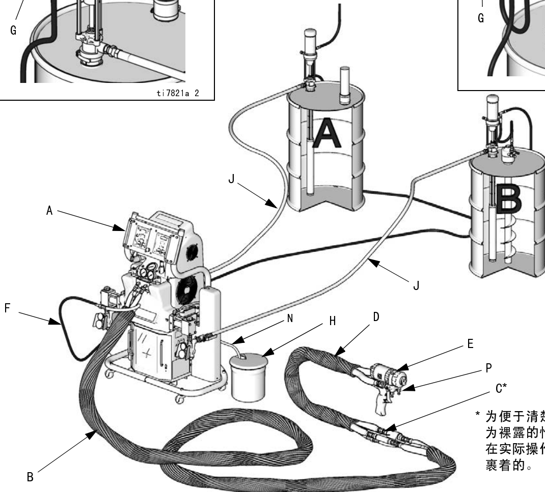
图 2. 典型安装，不带循环
