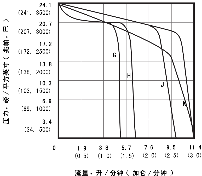
涂层喷涂性能表
