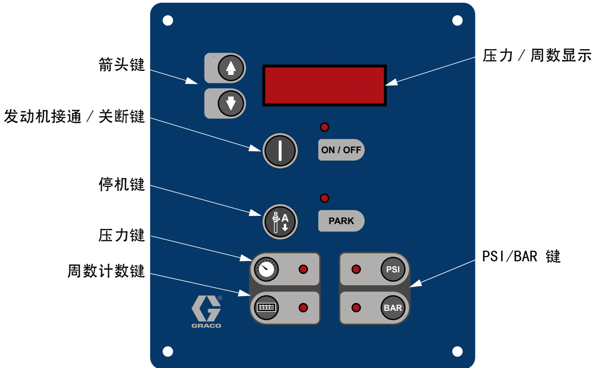
图 5. 发动机控制器及指示灯
