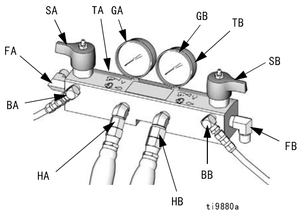
图 3. 组件识别 ( 所示型号为 H40 15.3 千瓦 )
