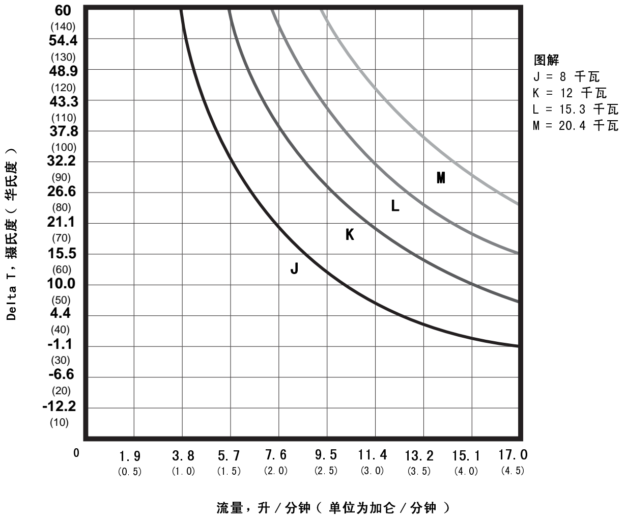
加热器性能表
