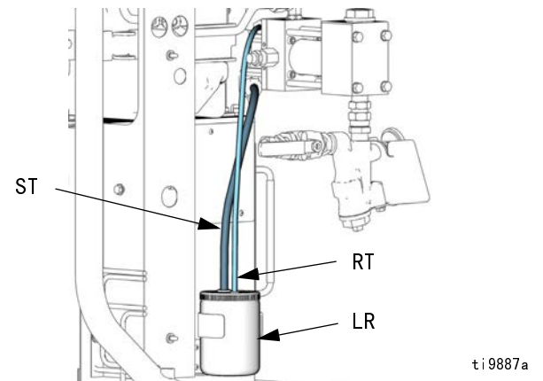
图 7. 泵润滑系统
