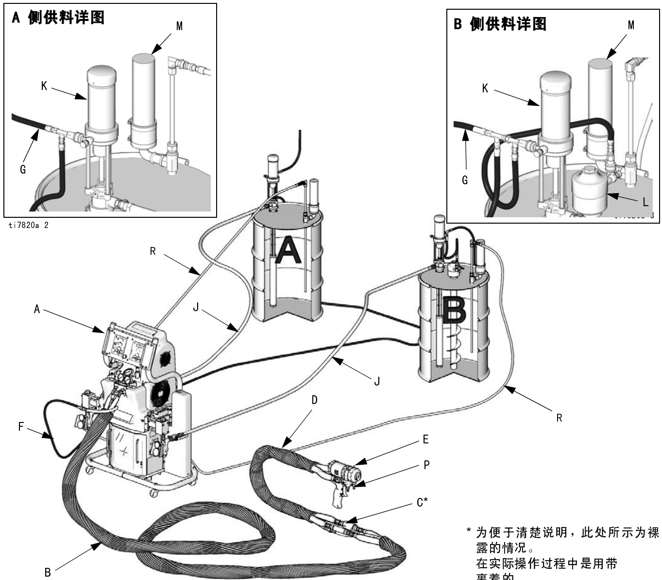
图 1. 典型安装，带循环
