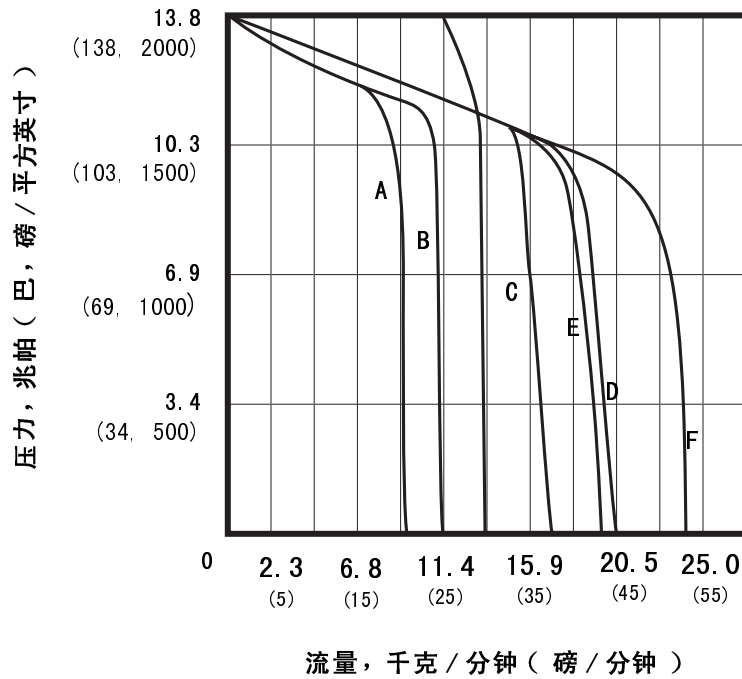
泡沫喷涂性能表
