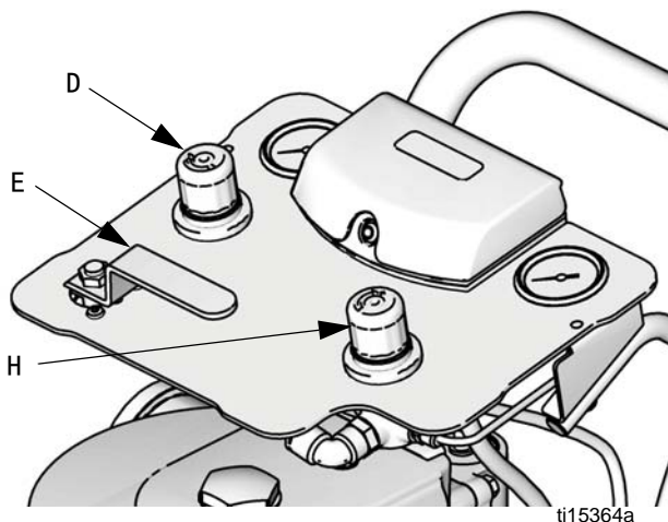
图 6. 气流控制器
