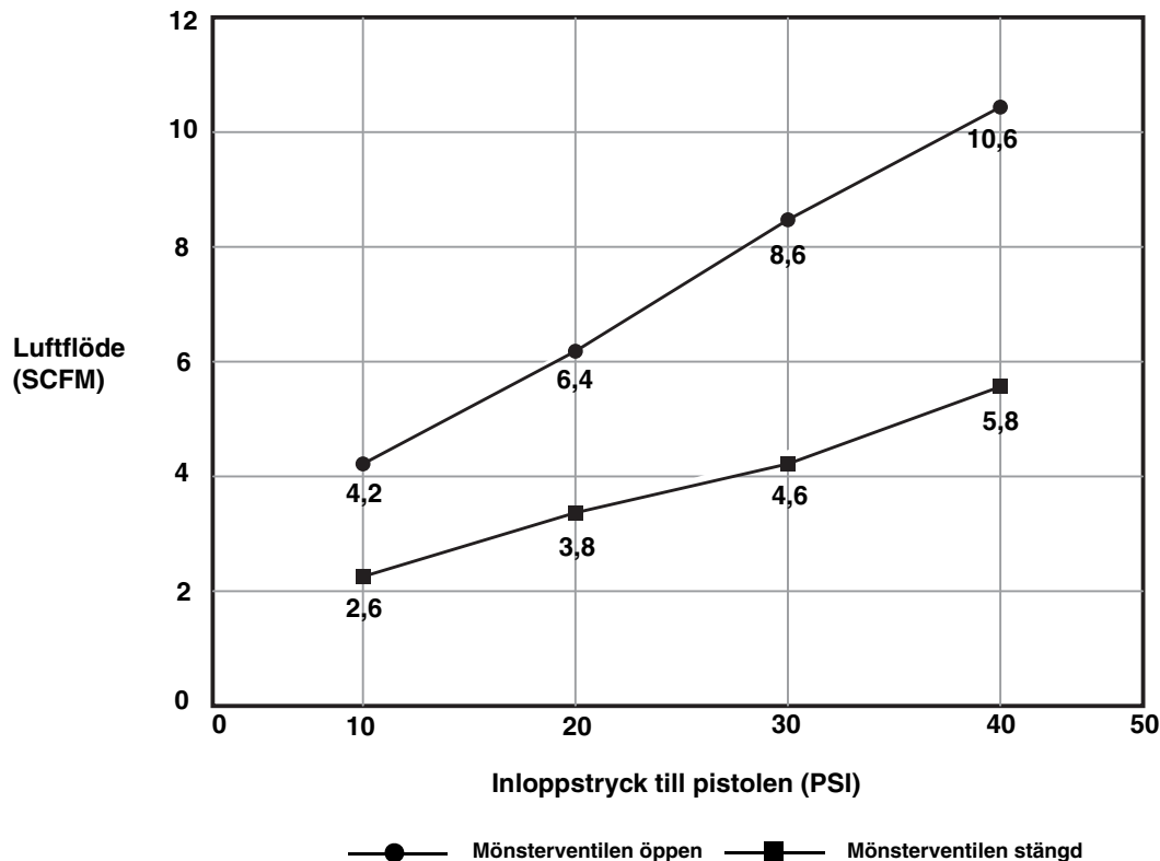
Air Flow, standard luftmunstycke för AA-serien
