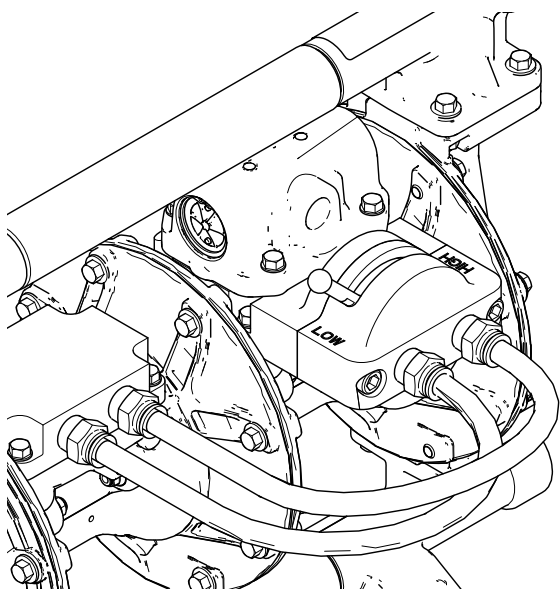
Figure 4 Hoog-/laagdrukhefboom
