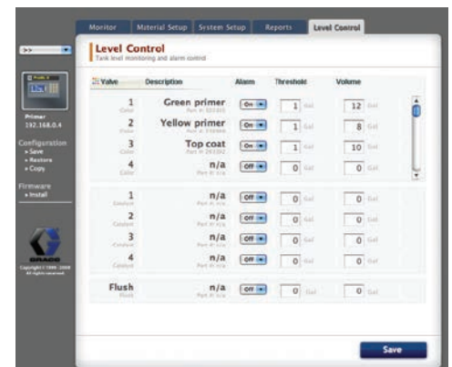
Gelişmiş İnternet Arayüzü ekran görüntüsü
