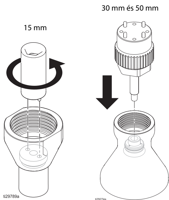
ÁBRA 19. Ütközőlap eltávolítása
