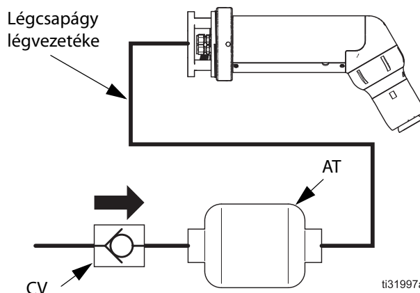
ÁBRA 8 A légcsapágy táplevegőjét biztosító vezeték légygújtó kamrával és visszacsapó szeleppel
