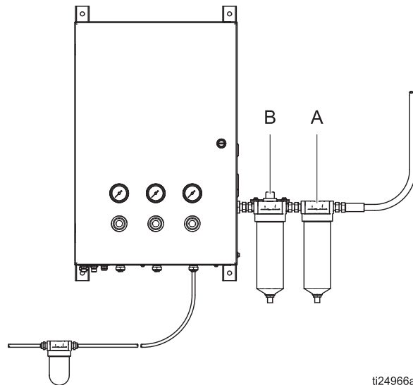
ÁBRA 7. Légszűrők
