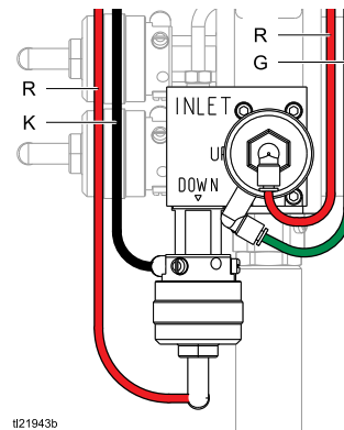
Figure 20 Conexiones de los tubos del colector de entrada
