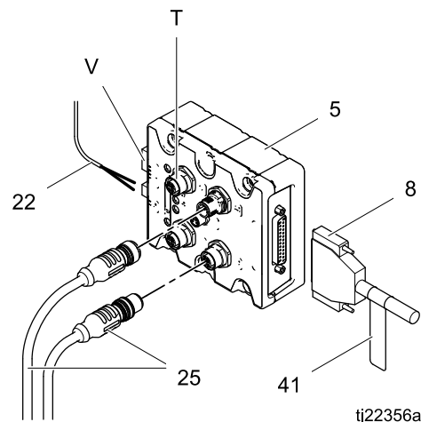
Figure 25 Conexiones del módulo de control de bomba
