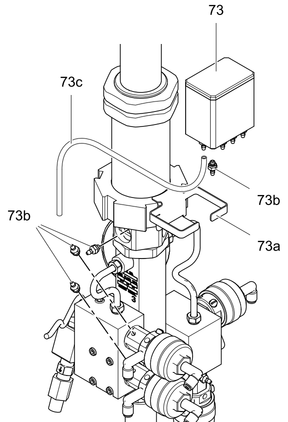
Figure 4 Instalación del kit de recipiente TSL
