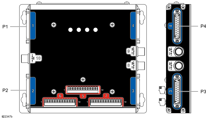
Figure 9 Puntos de conexión del módulo de control de fluido mejorado
