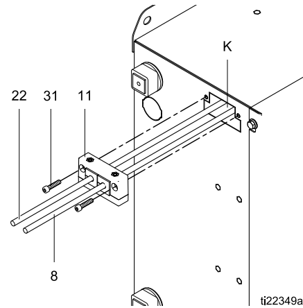
Figure 8 Instalación del ojo en la caja de control eléctrico
