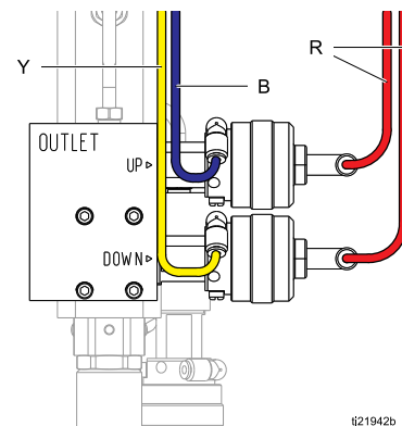
Figure 22 Conexiones de los tubos del colector de salida
