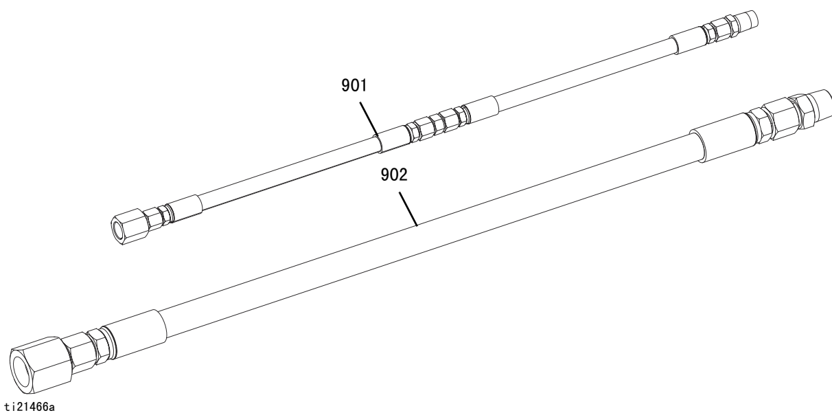
図 13: ホースキット
