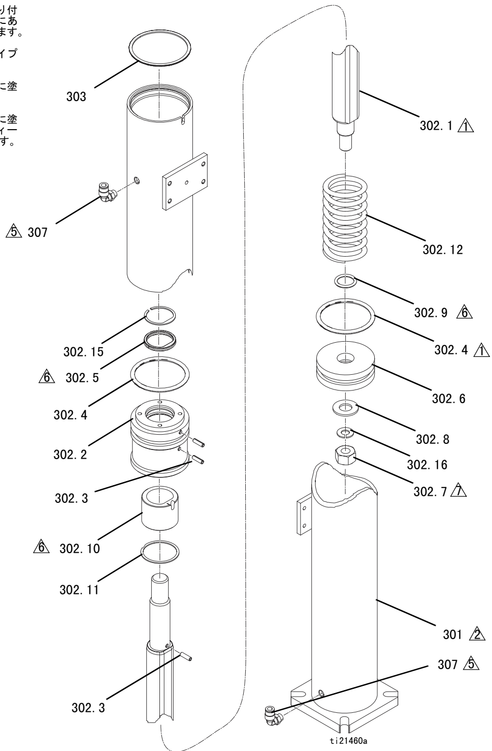
図 6: 18.9 リットル (5 ガロン) エアシリンダ
