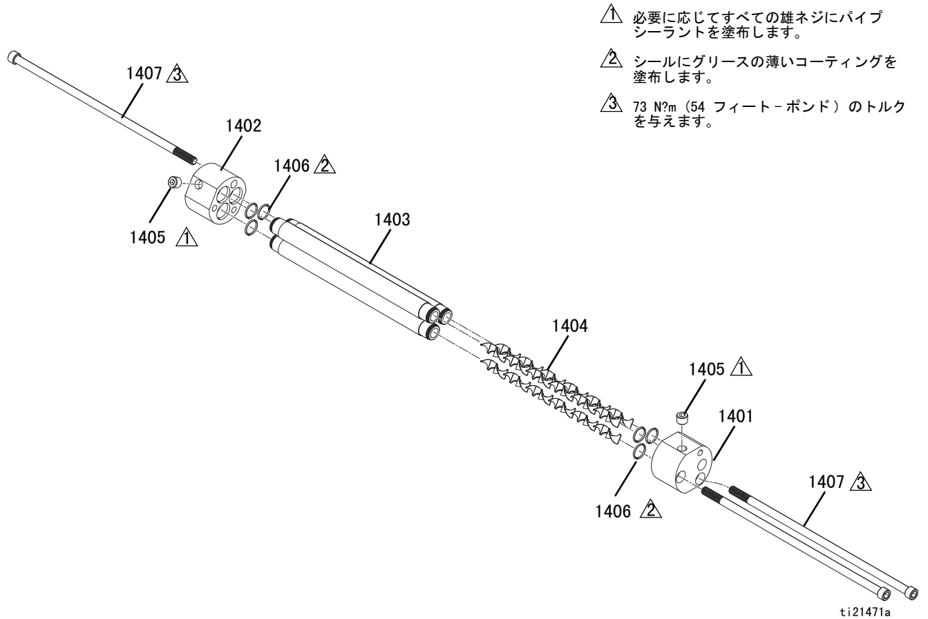
図 17: Tri-Core ミキサー
