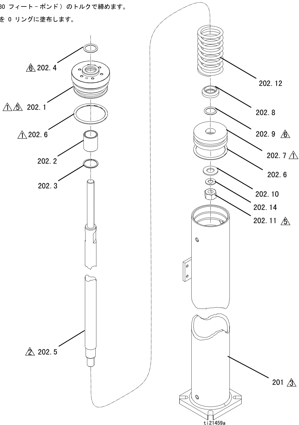
図 5: 208 リットル (55 ガロン) エアシリンダ
