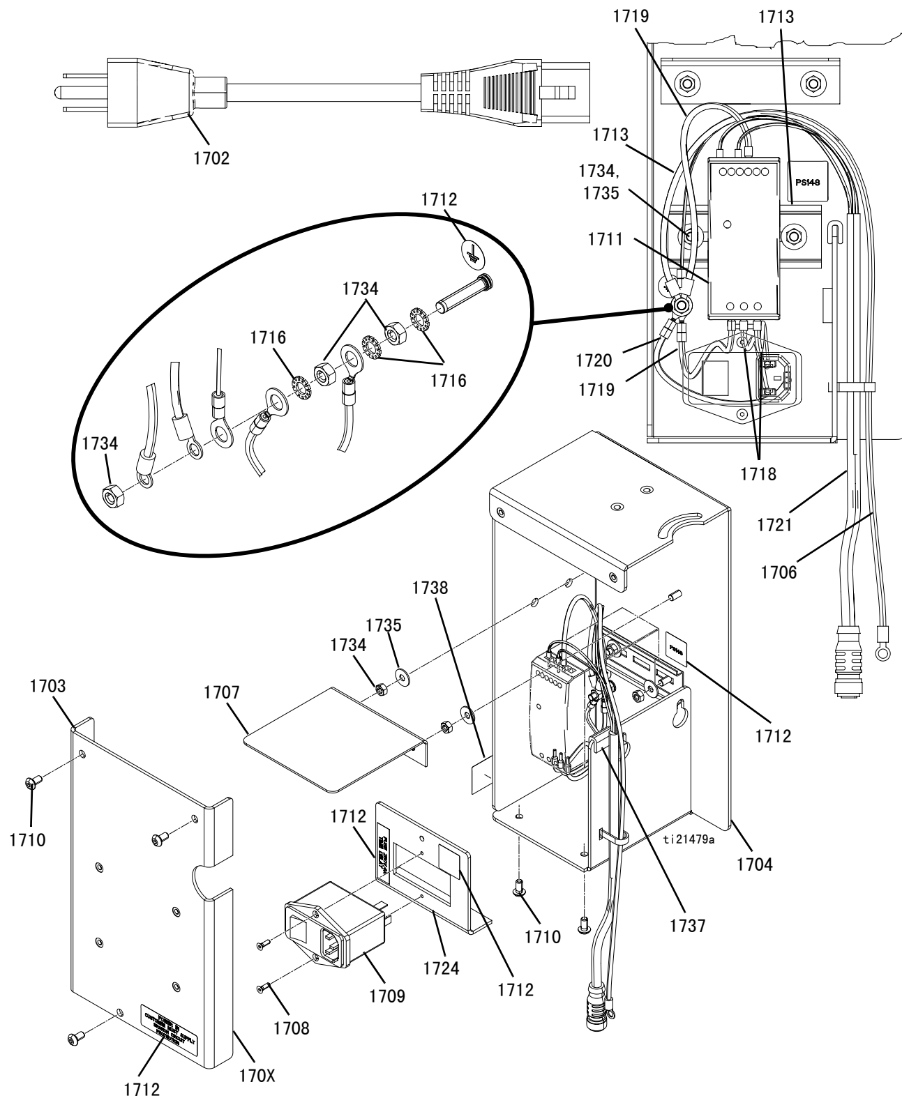
図 7: 電気エンクロージャ
