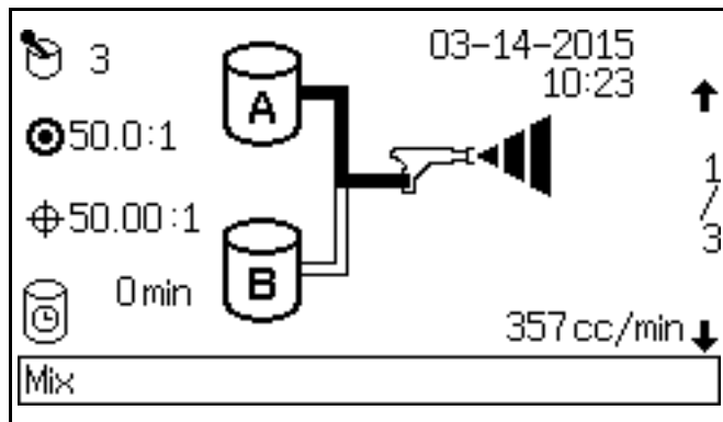
그림 62. 상태 화면
