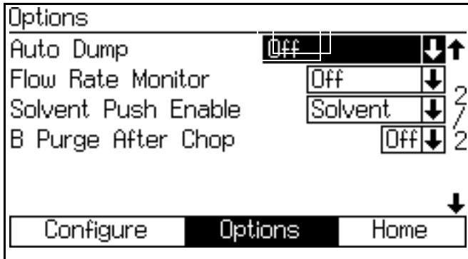
그림 31. 옵션 화면 2
