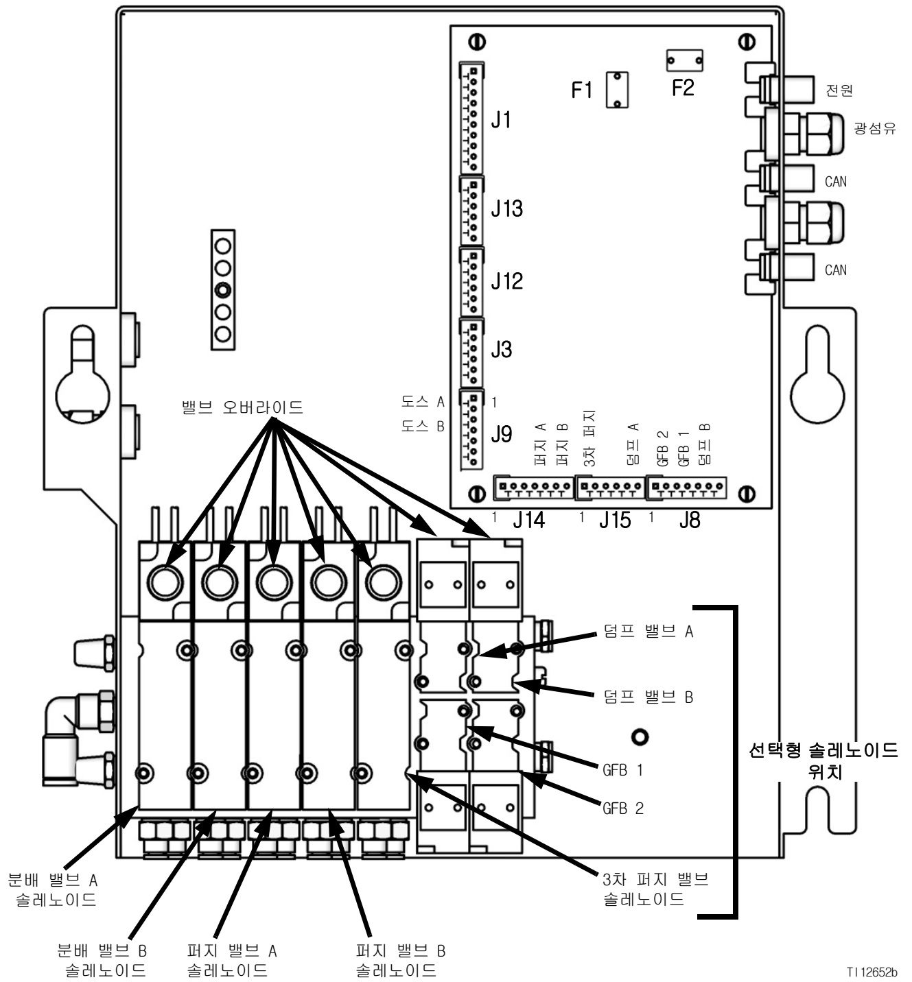
그림 65. 유체 솔레노이드
