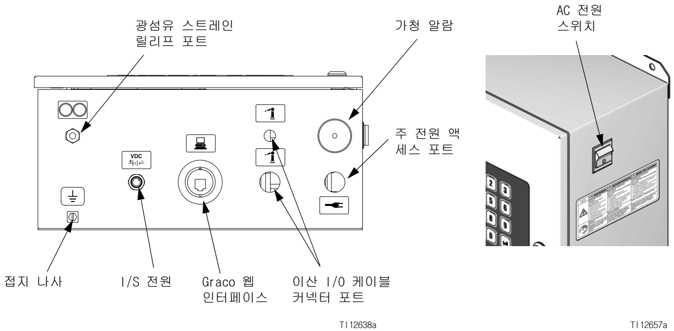
그림 6. EasyKey 연결 및 AC 전원 스위치
