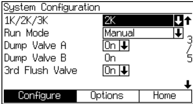
그림 24. 구성 화면 3
