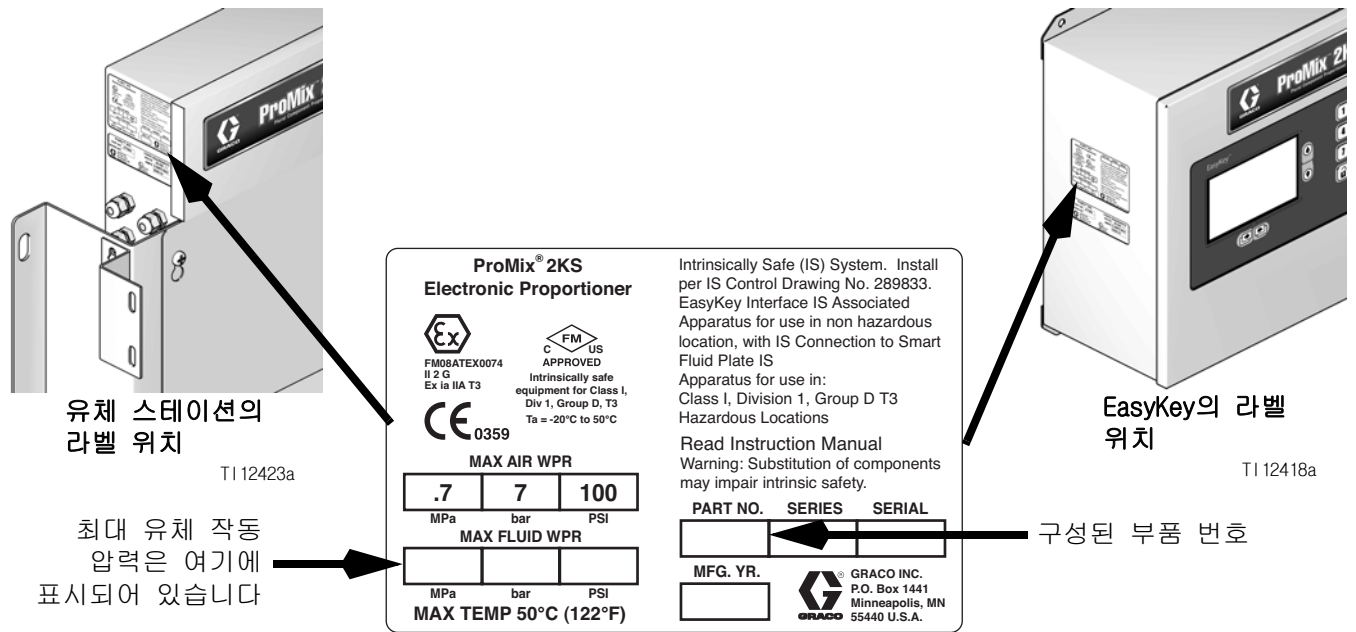
그림 1: 식별 라벨
