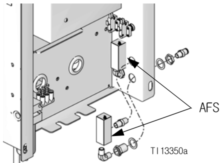
그림 60: 공기 흐름 스위치
