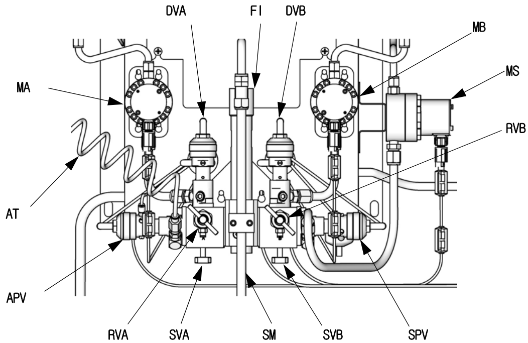
그림 3. 벽 장착형 유체 스테이션
