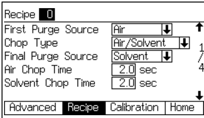
그림 46. 레서피 0 화면 1
