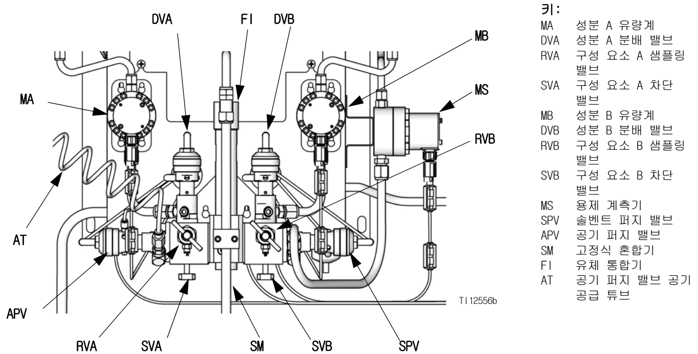
그림 67. 벽 장착형 유체 스테이션
