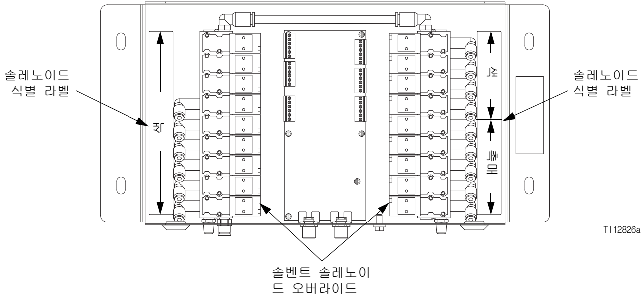
그림 66: 색 변경 솔레노이드
